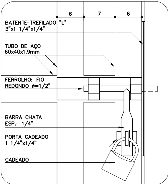
DETALHE 4B ESC. 1:5
