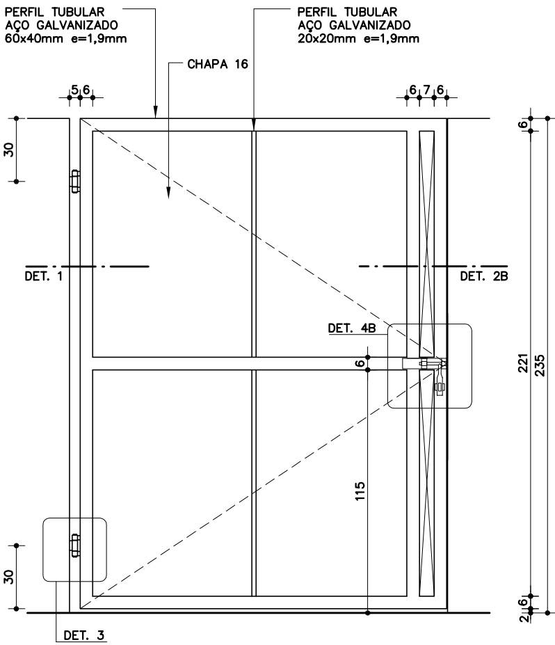
VISTA INTERNA PT-42 ESC. 1: 25
