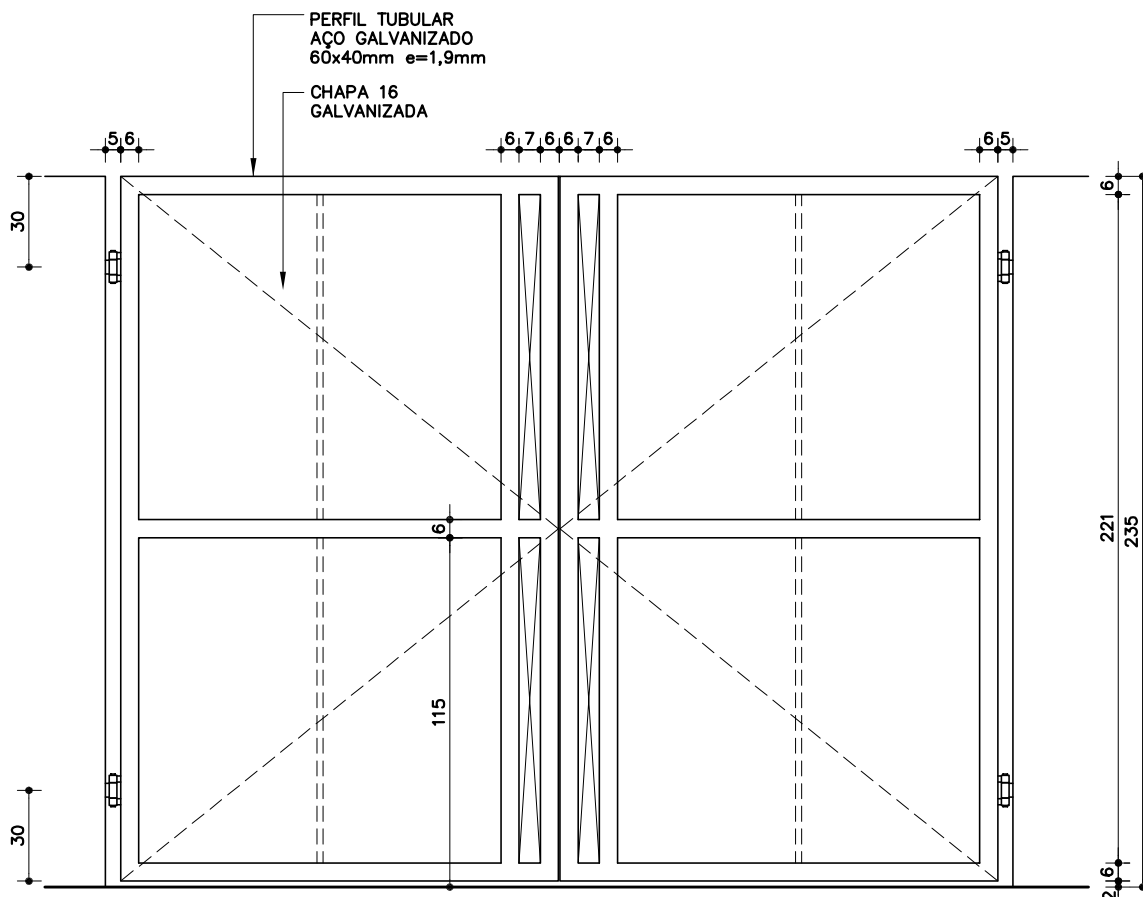
VISTA EXTERNA PT-41 ESC. 1:25
