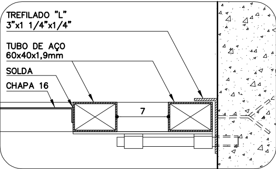
DETALHE 2A ESC. 1:5
