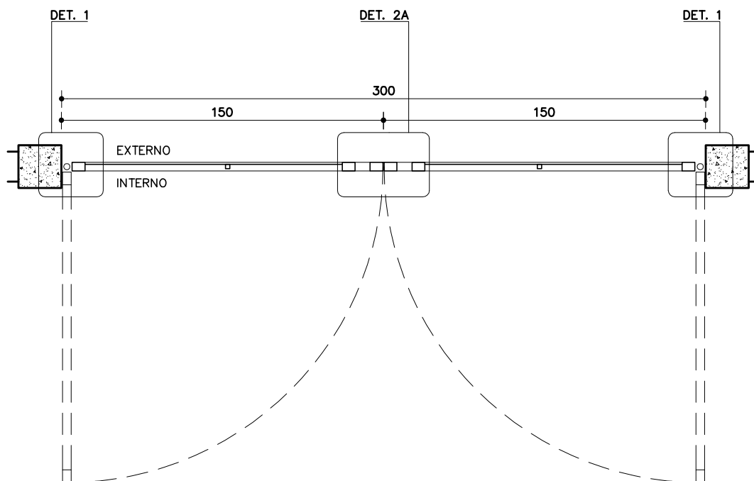
PLANTA PT-41
