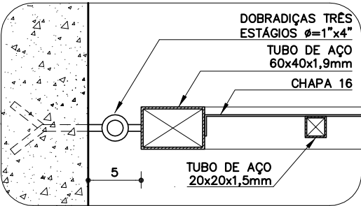
DETALHE 1 ESC. 1:5
