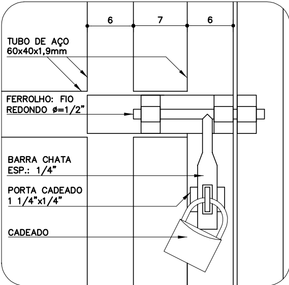
DETALHE 4A ESC. 1:5
