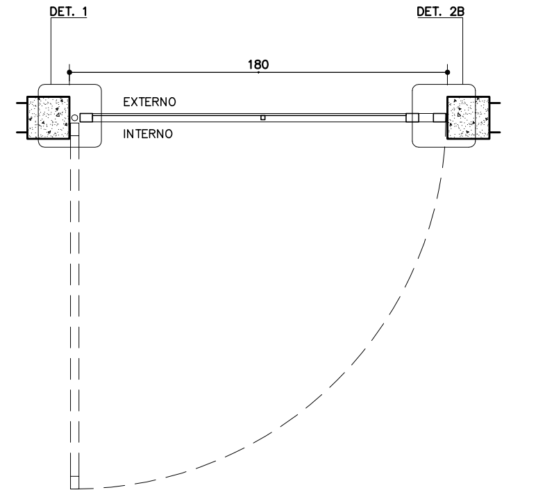
PLANTA PT-42 ESC. 1: 25
