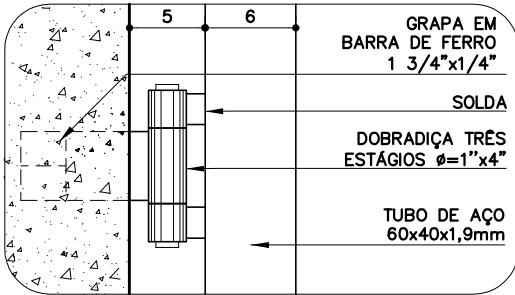
DETALHE 3 ESC. 1:5
