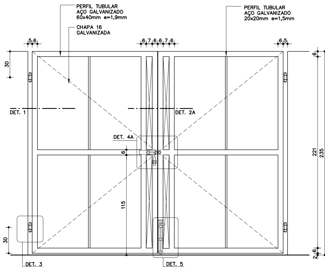
VISTA INTERNA PT-41
