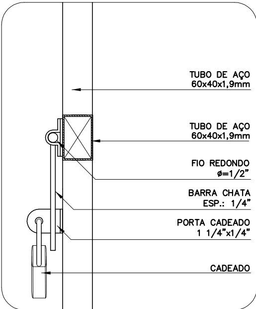
DETALHE 4A E 4B VISTA LATERAL ESC. 1:5
