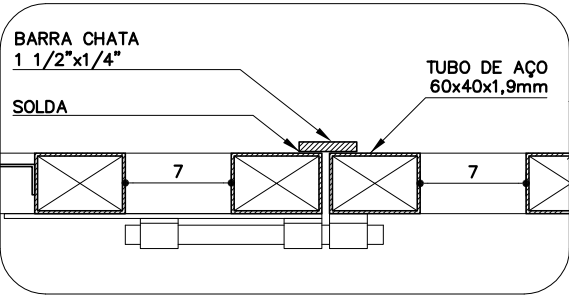
DETALHE 2A ESC. 1:5
