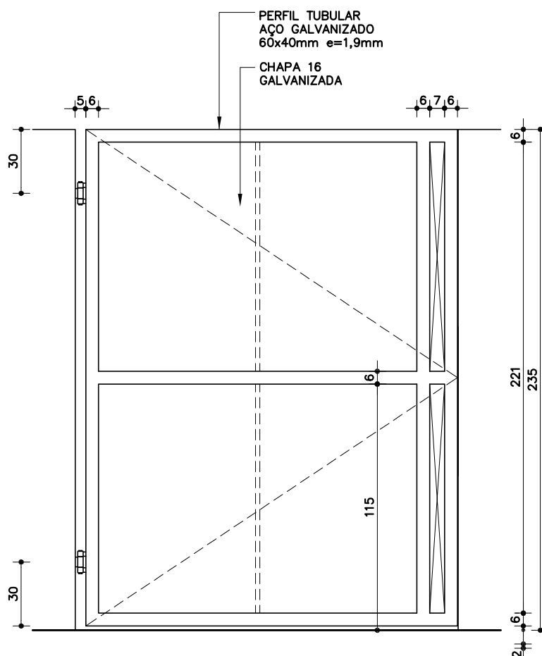
VISTA EXTERNA PT-42 ESC. 1:25
