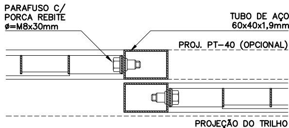
DETALHE 2 ESC. 1:5
