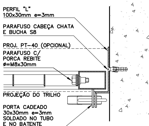
DETALHE 3 ESC. 1:5
