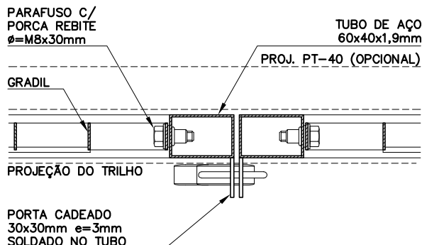
DETALHE 4 ESC. 1:5
