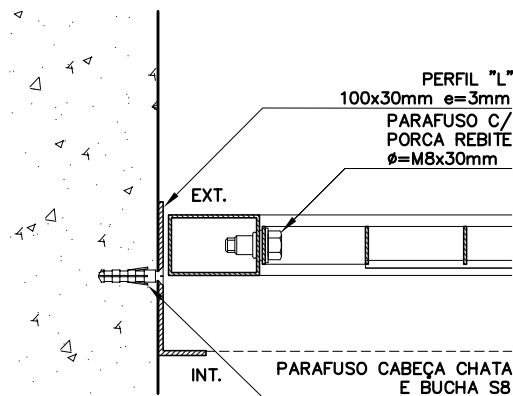
DETALHE 1 ESC. 1:5
