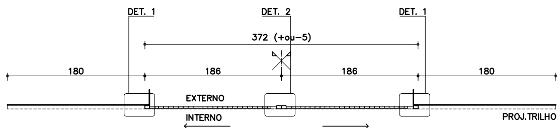
PLANTA PT-45
