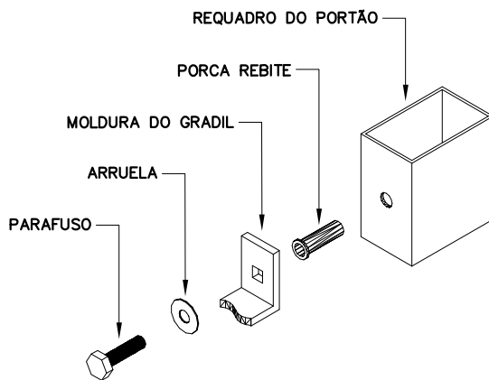
DET. FIXAÇÃO DO GRADIL
