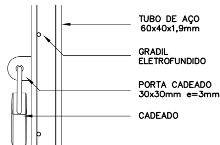
DET. PORTA CADEADO
