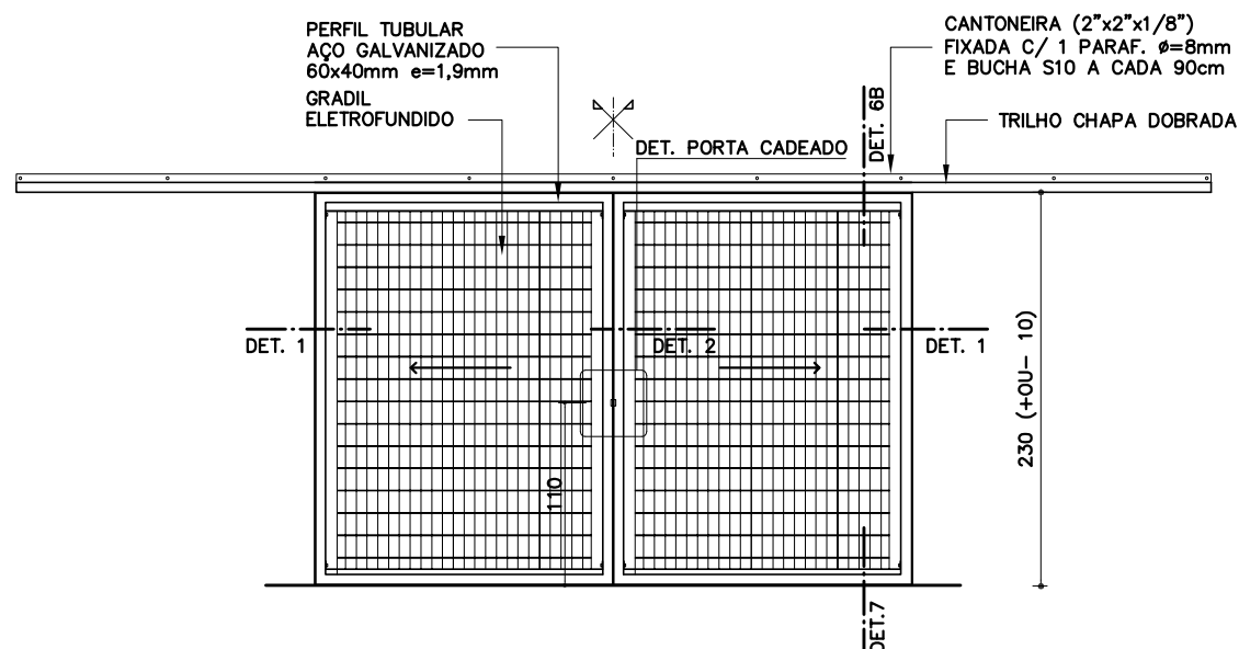
ELEVÇÃO INTERNA PT-45
