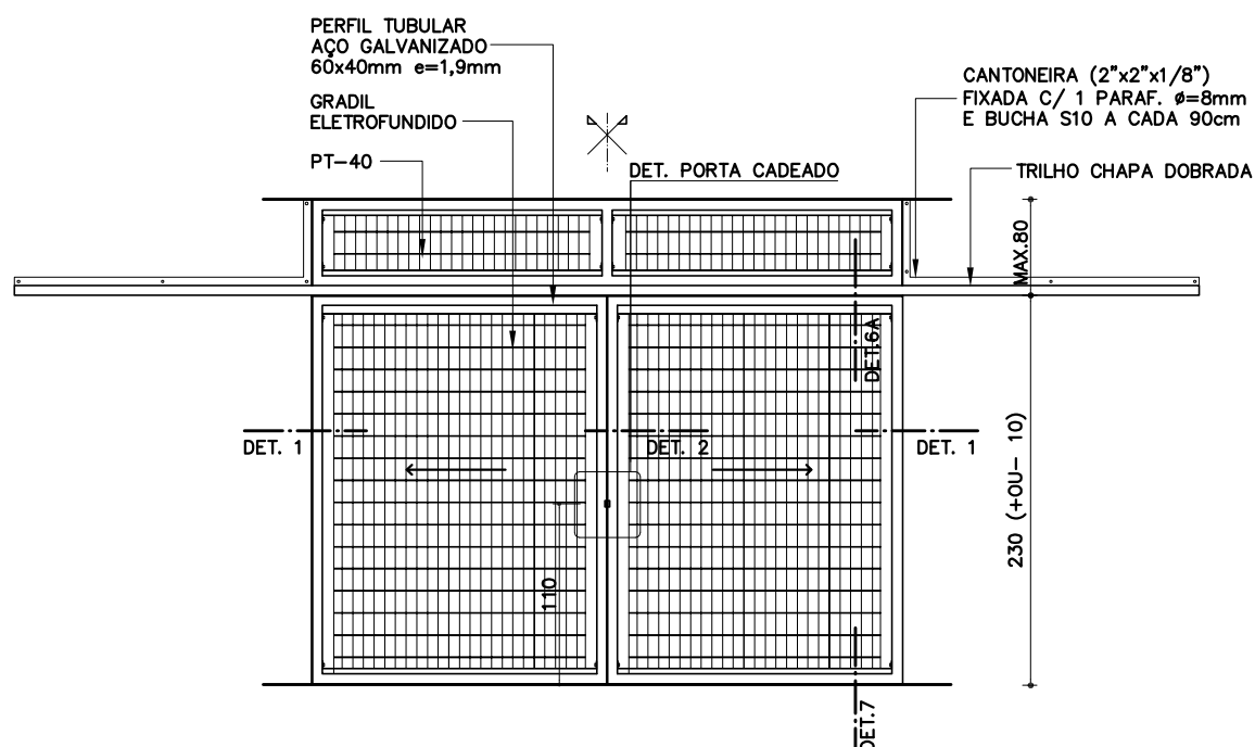
ELEVÇÃO INTERNA PT-45 COM PT-40
