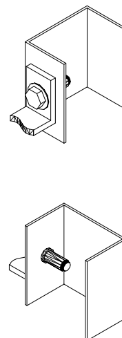
DET. PORTA CADEADO
