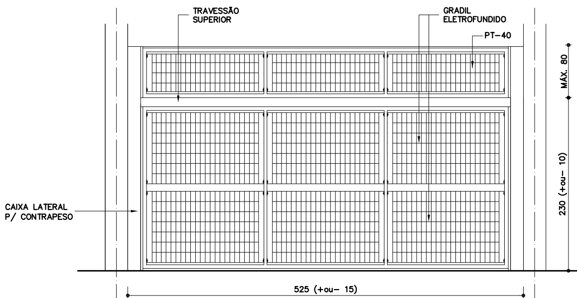
ELEVAÇÃO EXTERNA PT-48 COM PT-40
