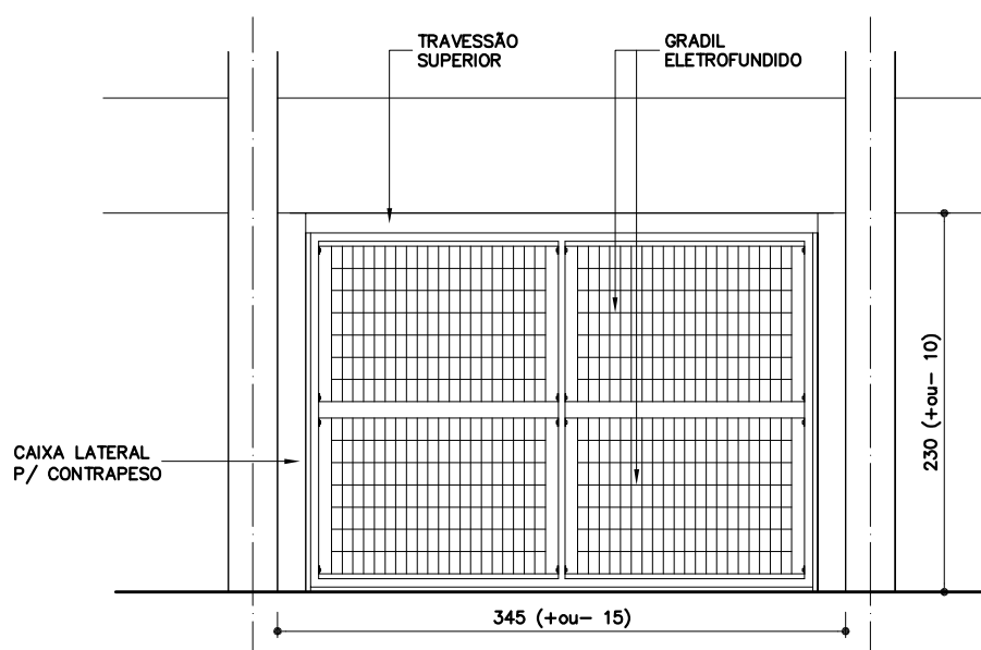
ELEVAÇÃO EXTERNA PT-49 ESC. 1: 50
