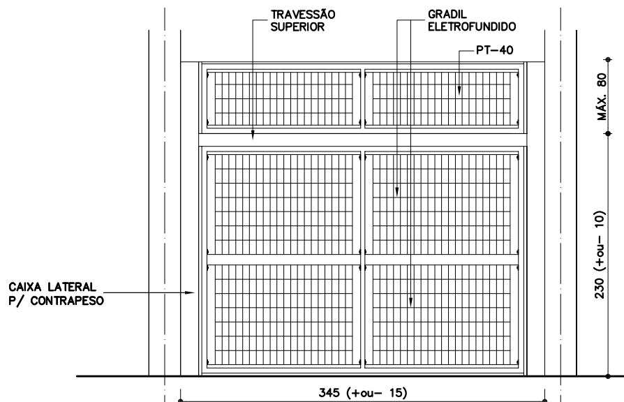
ELEVAÇÃO EXTERNA PT-49 COM PT-40
