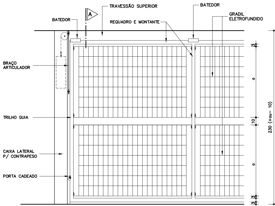
AMPLIAÇÃO PARCIAL – VISTA INTERNA ESC. 1:25
