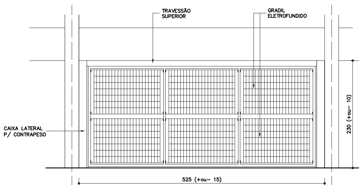
ELEVAÇÃO EXTERNA PT-48 ESC. 1: 50
