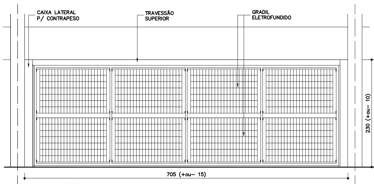
ELEVAÇÃO EXTERNA PT-47 ESC. 1: 50
