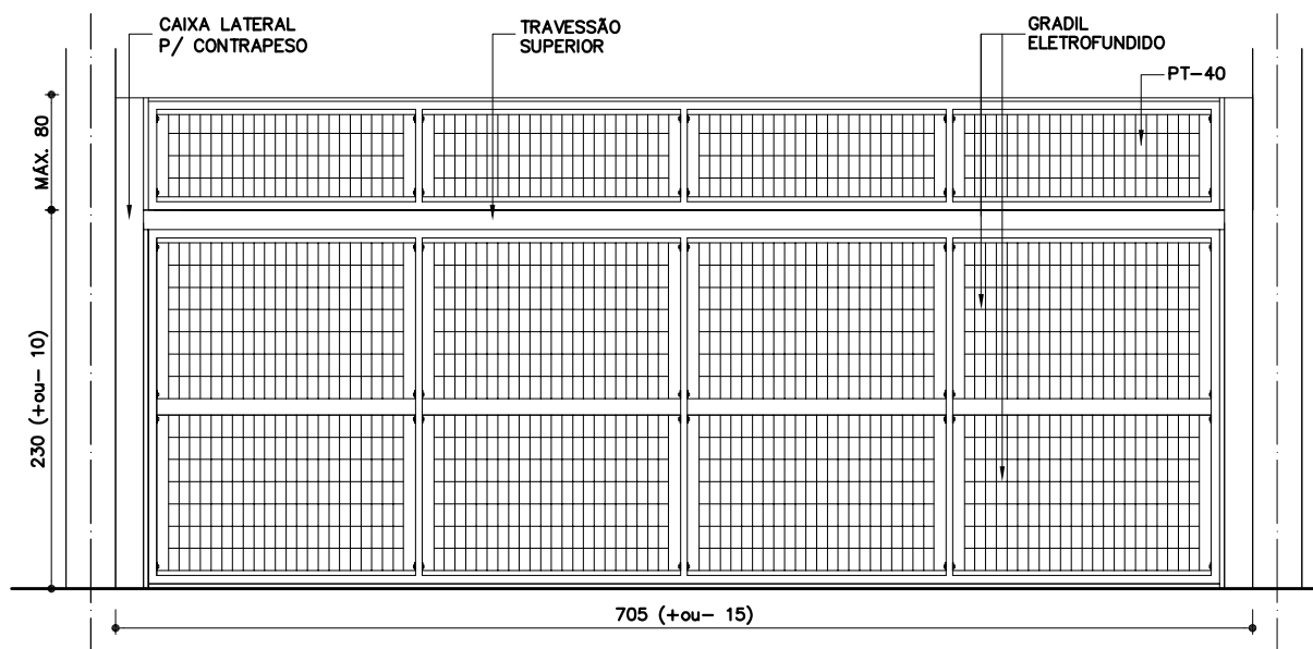
ELEVAÇÃO EXTERNA PT-47 COM PT-40
