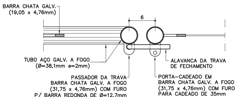
DETALHE 2 ESC. 1:5
