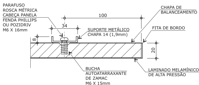
CORTE LONGITUDINAL
