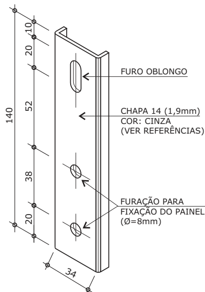
SUORTE METÁLICO
