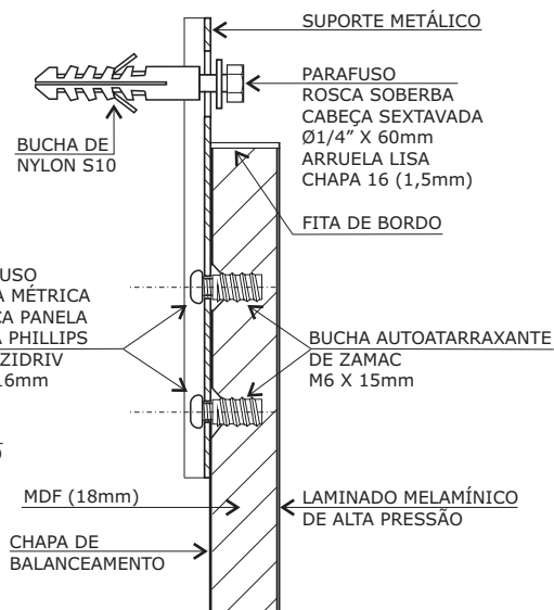
CORTE TRANSVERSAL
