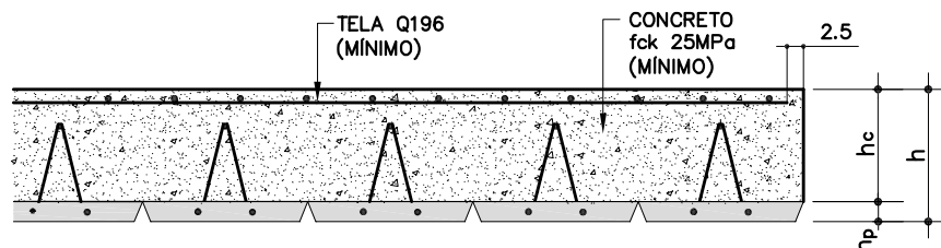
PERÍMETRO DO PISO (P) PRÉ-LAJE TRELIÇADA MACIÇA
