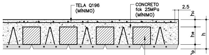
PERÍMETRO DO PISO (P) PRÉ-LAJE TRELIÇADA COM ELEMENTOS INERTES
