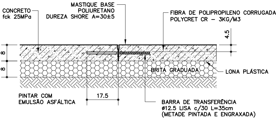
JUNTA DE CONSTRUÇÃO (C)
