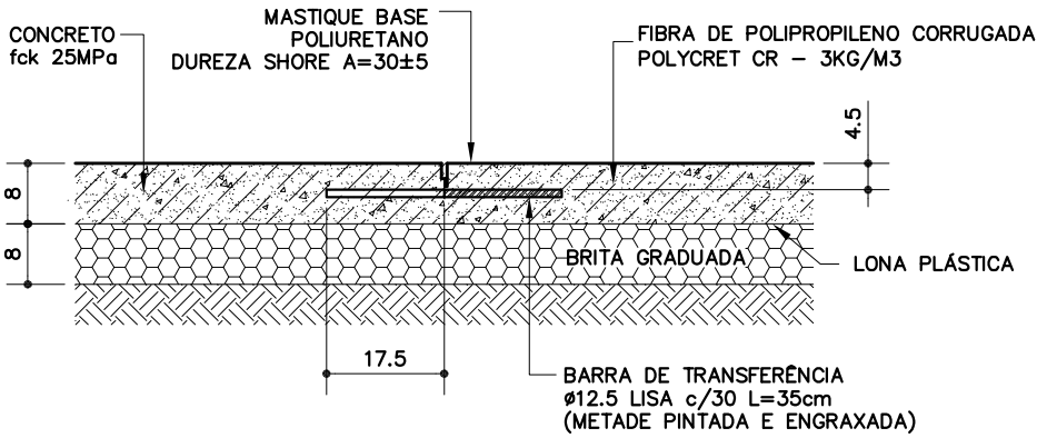
JUNTA SERRADA (S)
