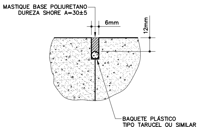
SELANTE PARA JUNTA DE CONSTRUÇÃO (C)
