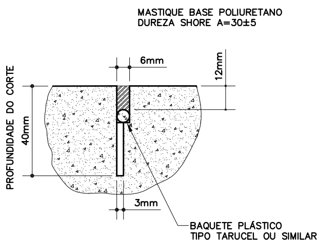
SELANTE PARA JUNTA SERRADA (S)
