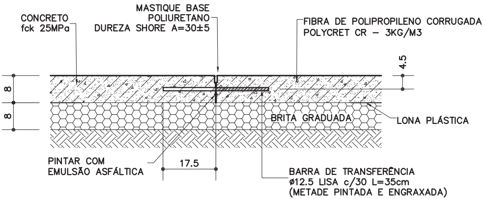
JUNTA DE CONSTRUÇÃO (C)
