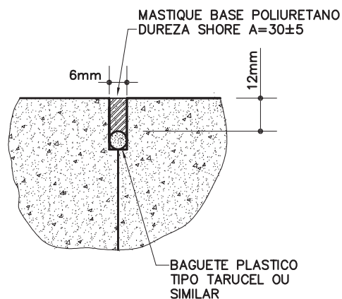
SELANTE PARA JUNTA DE CONSTRUÇÃO (C)
