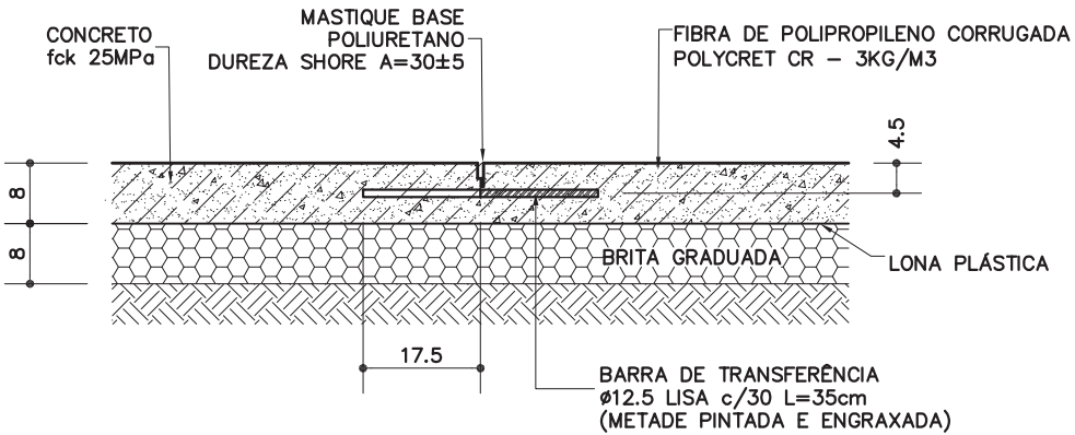
JUNTA SERRADA (S)
