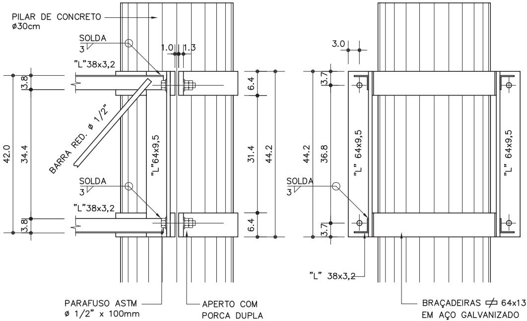
VISTA LATERAL
