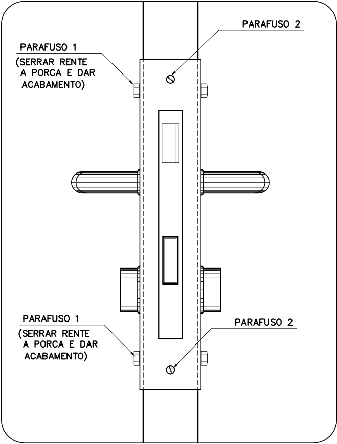
VISTA DO COMPONENTE APLICADO À PORTA ESC. 1: 2.5
