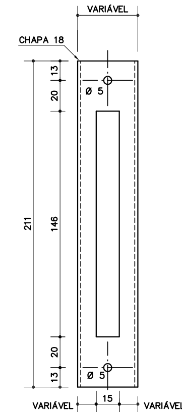
VISTA A CHAPA DOBRADA ESC. 1: 2.5
