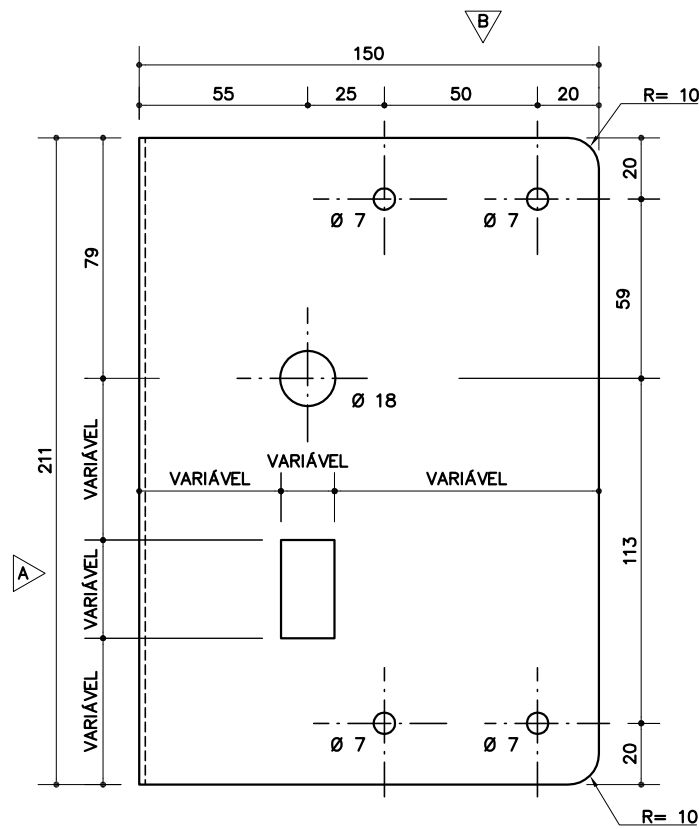
VISTA LATERAL CHAPA DOBRADA ESC. 1: 2.5
