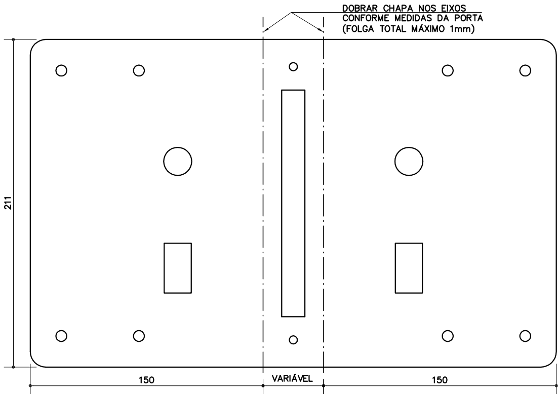
CHAPA ABERTA ESC. 1: 2.5
