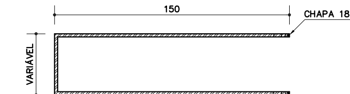
VISTA B - CHAPA DOBRADA ESC. 1: 2.5
