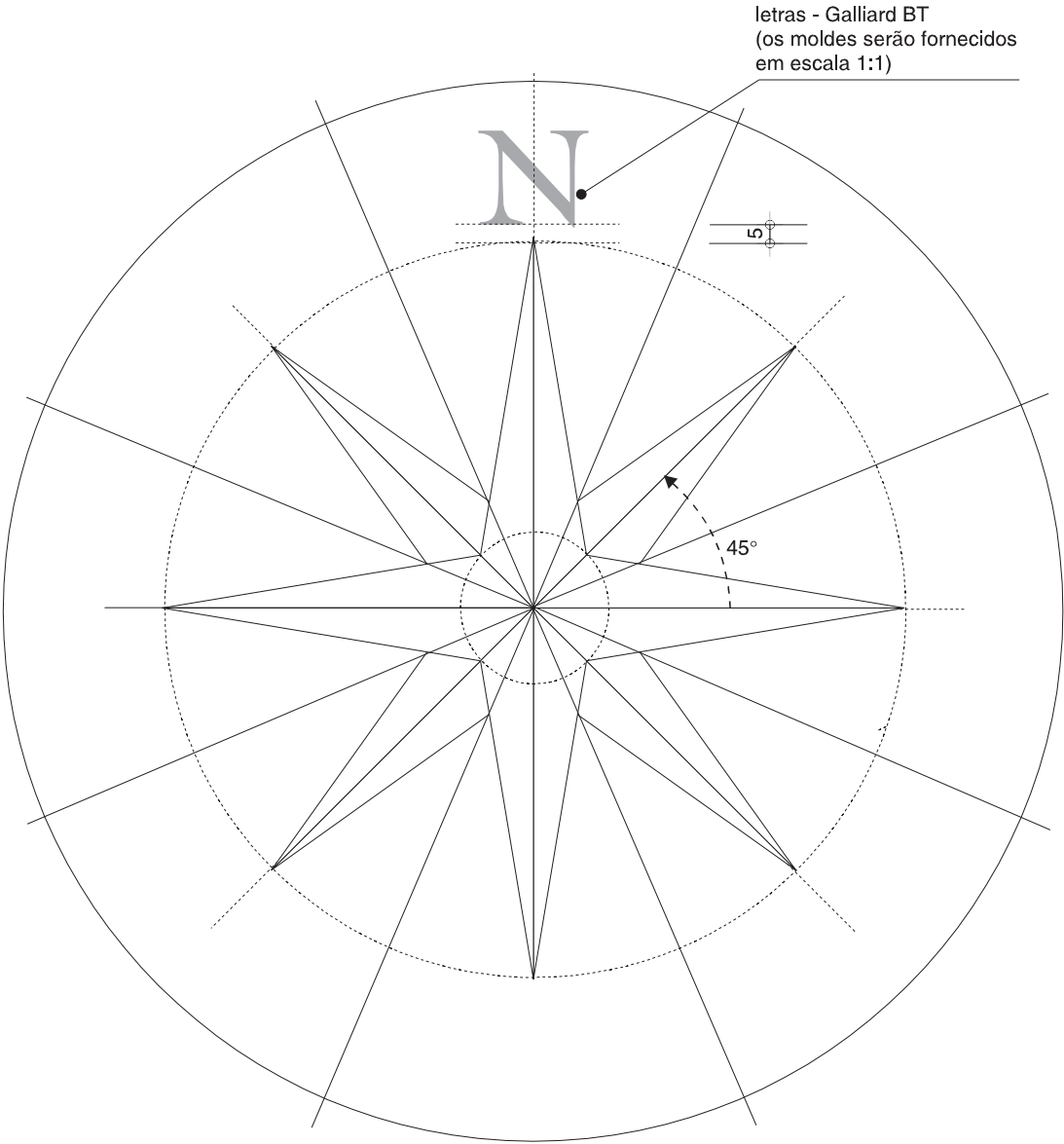
ESQUEMA CONSTRUTIVO esc. 1:25
