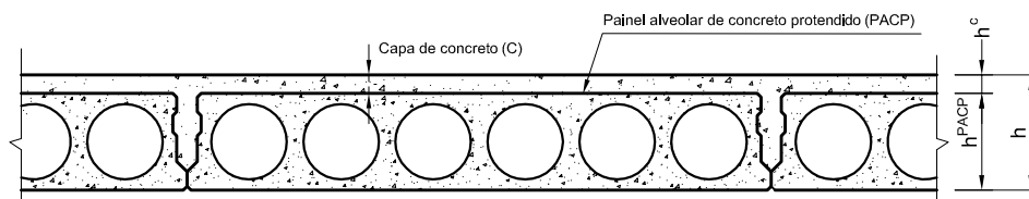
Laje pré-fabricada- Painel Alveolar de Concreto Protendido (PACP)
