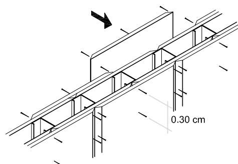
Figura - Divisória de Gesso Dupla
