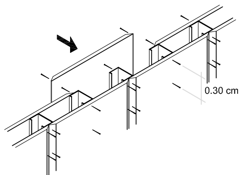
Figura - Divisória de Gesso Simples
