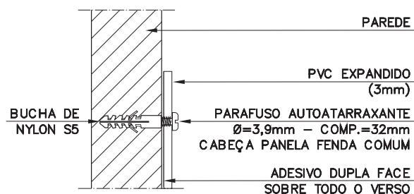
DETALHE DA FIXAÇÃO ESC.: 1:2
