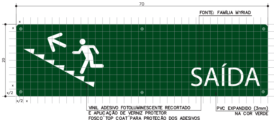
EXEMPLO ESC.: 1:5
