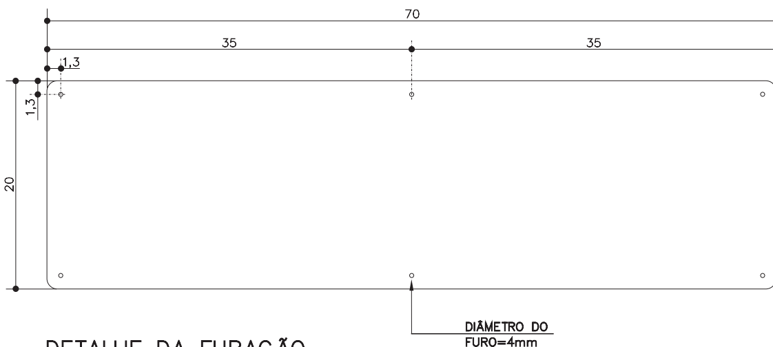
DETALHE DA FURAÇÃO ESC.: 1:5
