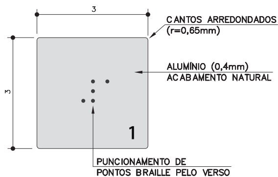
EXEMPLO ESC.: 1:1
