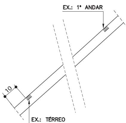
CHAPA METÁLICA APLICADA EM CORRIMÃO SEM PROLOGAMENTO SEM ESCALA
