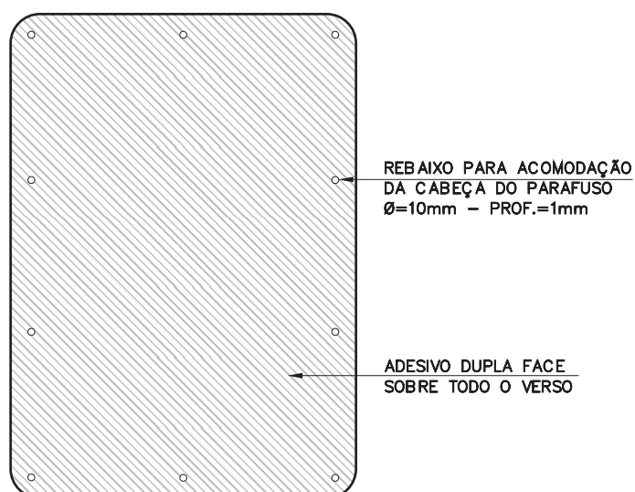
SUPERFÍCIE – FACE POSTERIOR DETALHE DO REBAIXO PARA ACOMODAÇÃO DA CABEÇA DO PARAFUSO ESC.: 1:10
