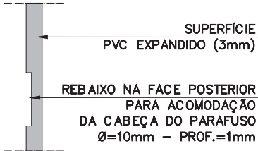
DETALHE FURAÇÃO NA SUPERFÍCIE ESC.: 1:1
