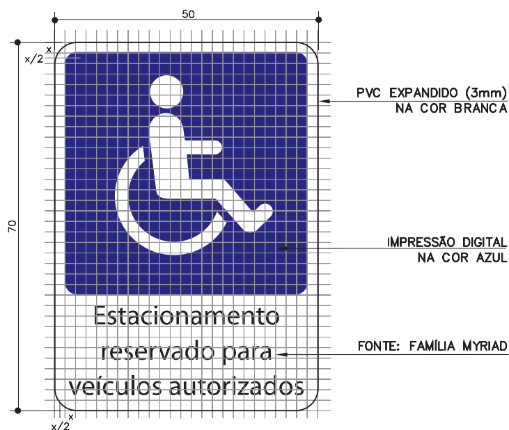
SUPERFÍCIE – FACE FRONTAL ESC.: 1:10
