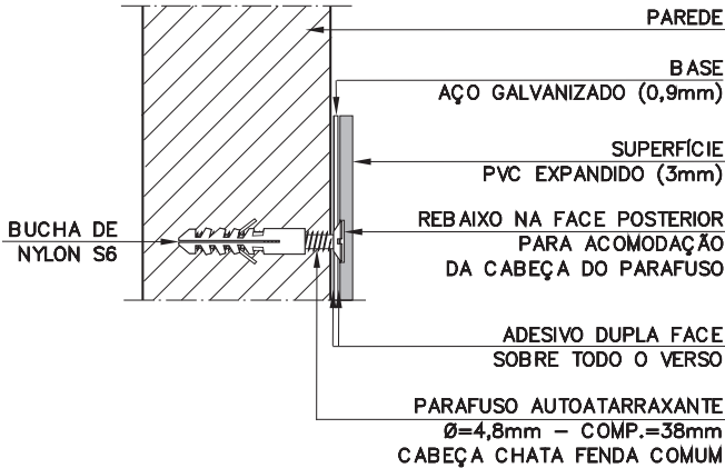
DETALHE DA FIXAÇÃO ESC.: 1:2
