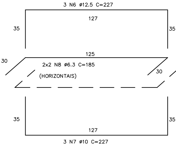
CORTE AA ESC. 1: 20
