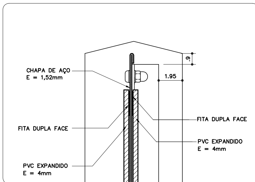
DETALHE 03 ESC. 1:2
