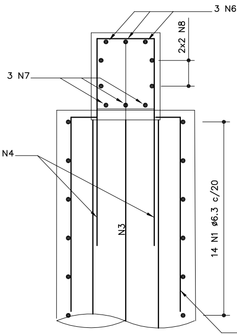
CORTE BB ESC. 1: 20
