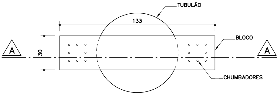
PLANTA ESC. 1: 20
