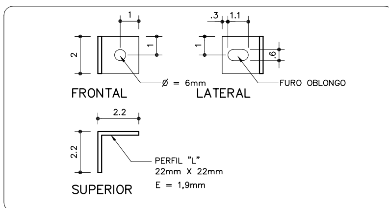
DETALHE DO SUPORTE
