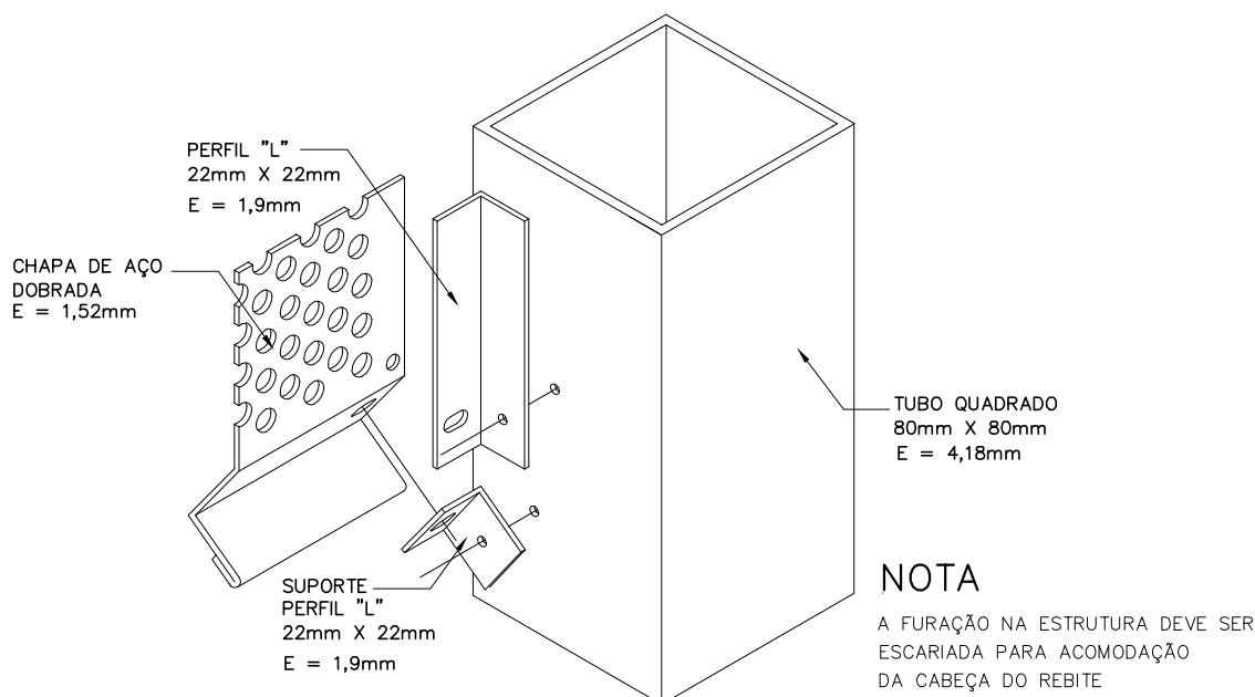
DET. DE FIXAÇÃO DA CHAPA (PARTE INFERIOR)
