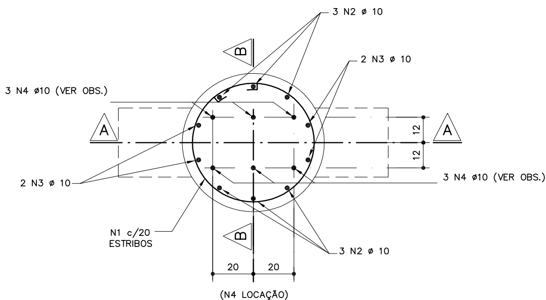
PLANTA— TUBULÃO ESC. 1:20
