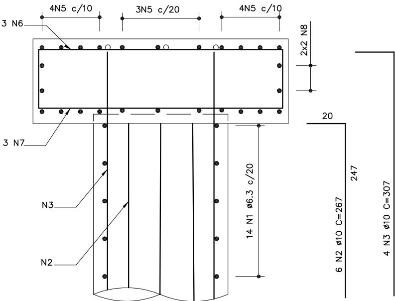
CORTE AA ESC. 1: 20
