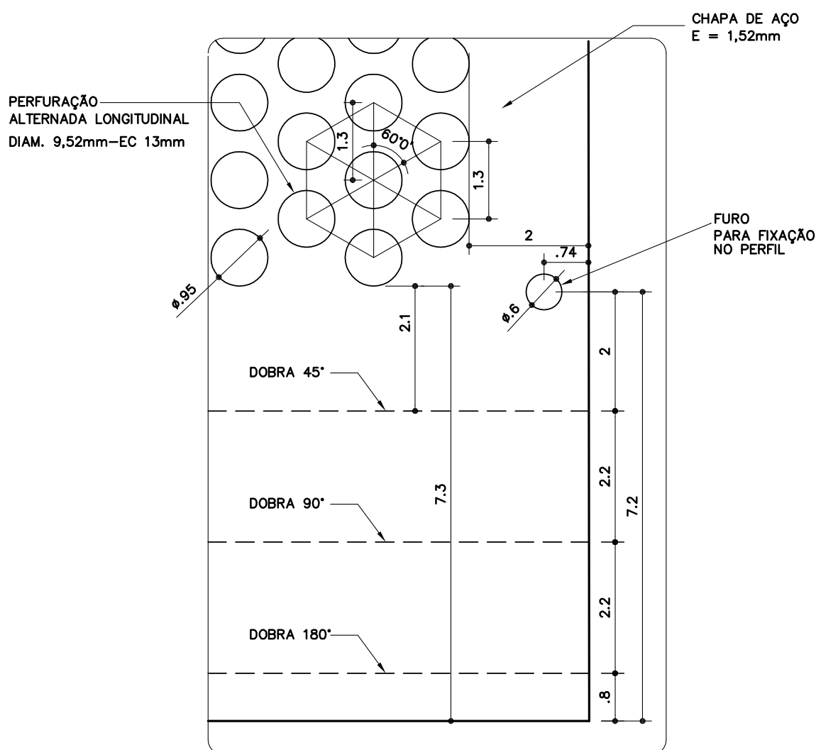
DETALHE 07 – CHAPA PLANIFICADA ESC. 1:1
