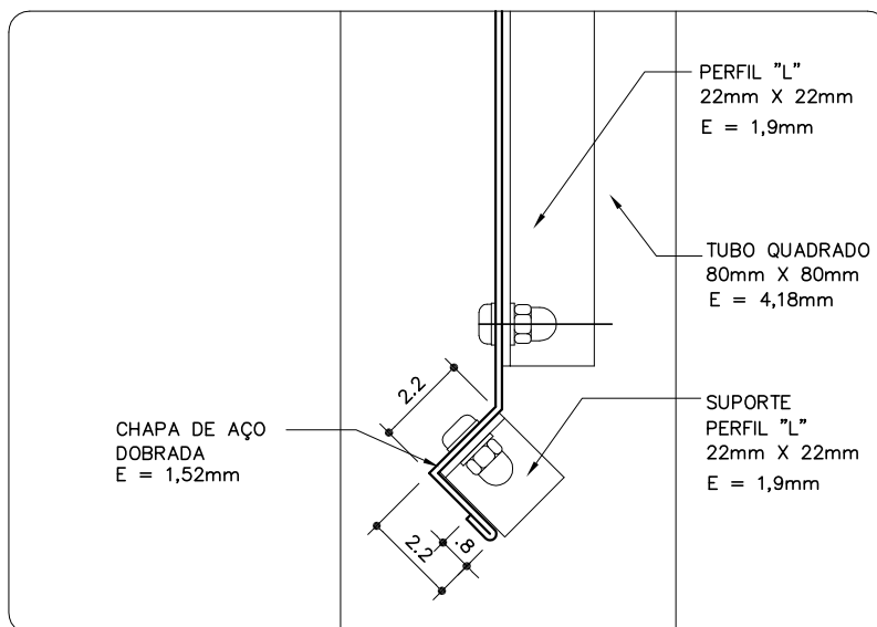
DETALHE 08
