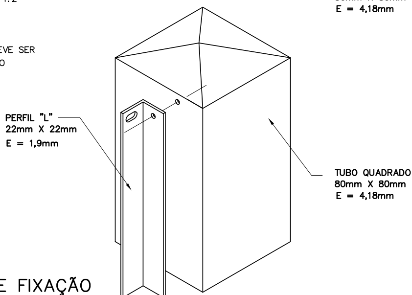
DETALHE 04 – VISTA POSTERIOR ESC. 1:2
