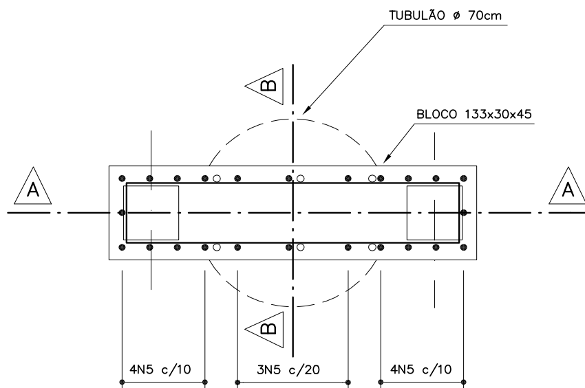
PLANTA— BLOCO ESC. 1:20
