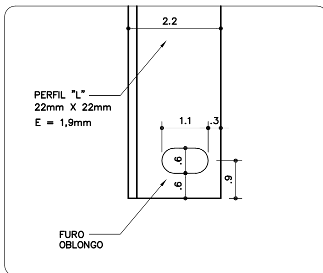
DETALHE 06 – PERFIL ESC. 1:1
