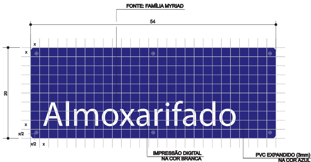
EXEMPLO APLICAÇÃO SOBRE PAINÉIS / PORTAS ESC.: 1:5
