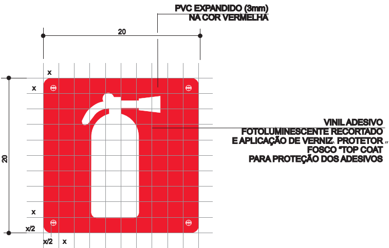
EXEMPLO ESC.: 1:5
