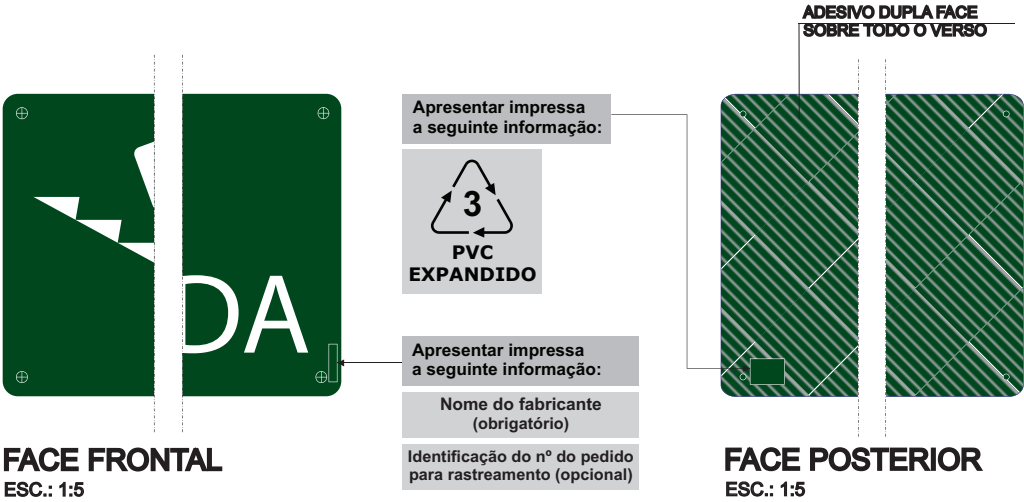
EXEMPLO ESC.: 1:5
