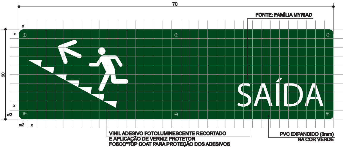
EXEMPLO ESC.: 1:5
