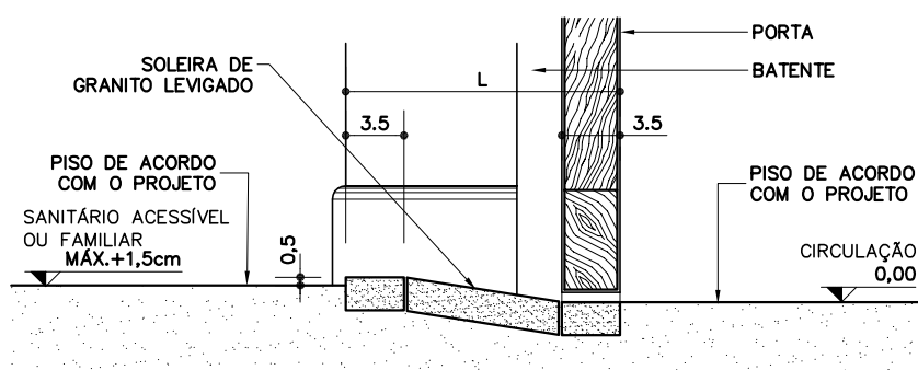
CORTE AA ESC. 1:5
