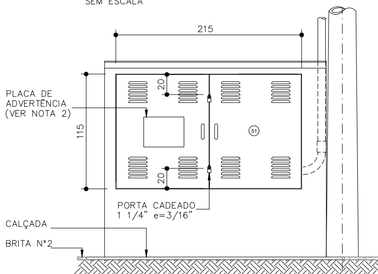
PORTA EXTERNA SEM ESCALA
