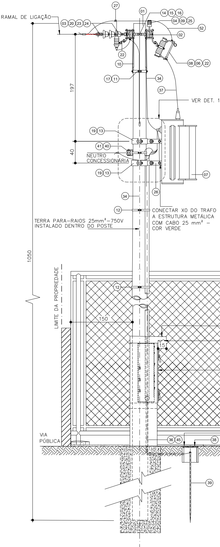
VISTA LATERAL SEM ESCALA
