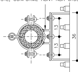
CORTE A SEM ESCALA
