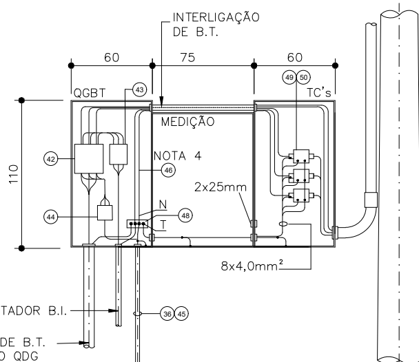
MONTAGEM INTERNA SEM ESCALA
