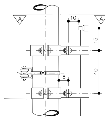
DETALHE 1 VISTA SEM ESCALA
