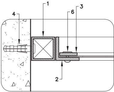
DET. 1 ESC. 1:2.5
