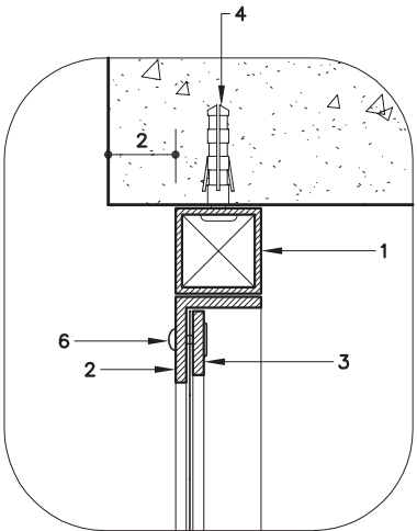
DET. 3
