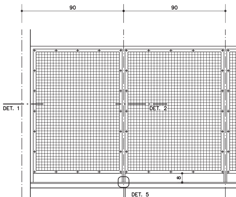
VISTA EXTERNA
