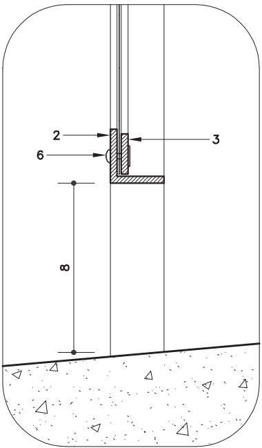
DET. 4
