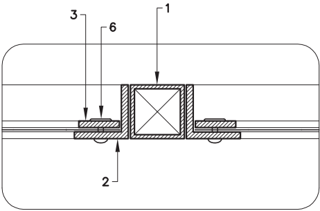
DET. 2
