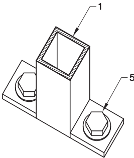
DET. 5
