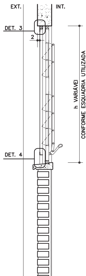
CORTE AA
