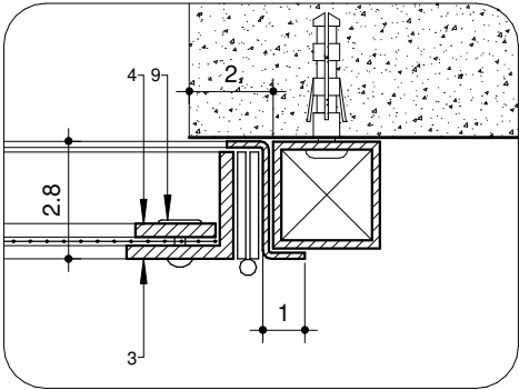
DET. 7 ESC: 1 : 2
