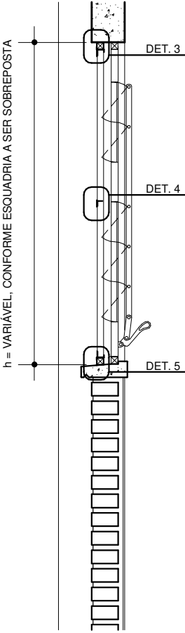
CORTE AA ESC: 1 : 20
