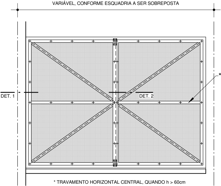
VISTA EXTERNA ESC: 1 : 20
