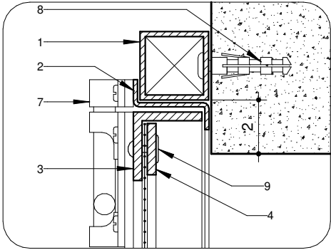
DET. 8 ESC: 1 : 2
