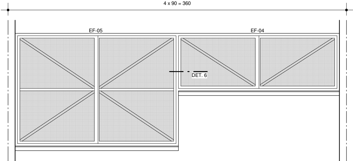
EXEMPLO DE ACOPLAMENTO SOBRE EF-05 E EF-04 ESC: 1 : 25
