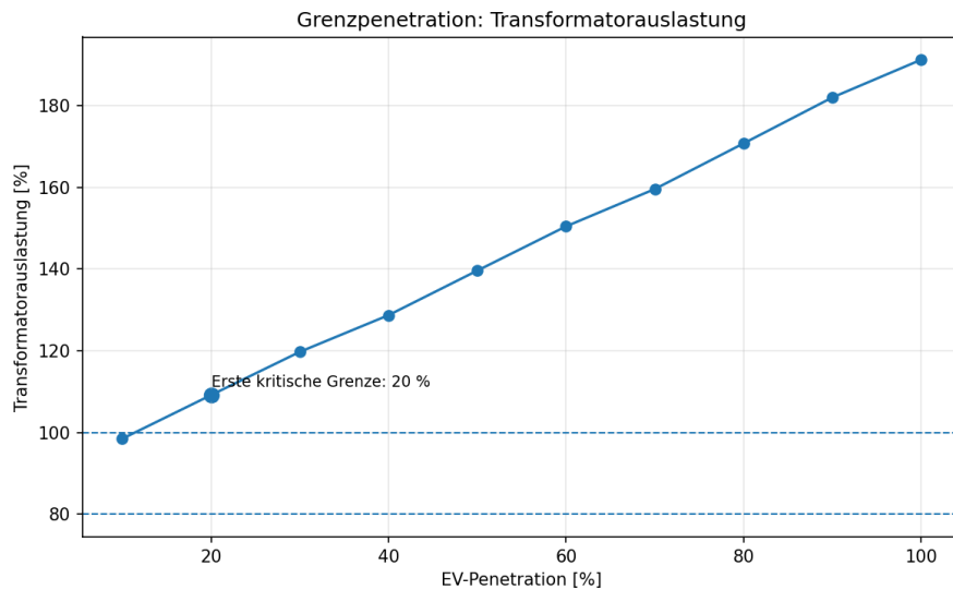
Abbildung 2: Grenzpenetration in Bezug auf die Transformatorauslastung.
