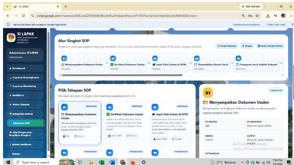
Gambar 31. Tahapan SOP
