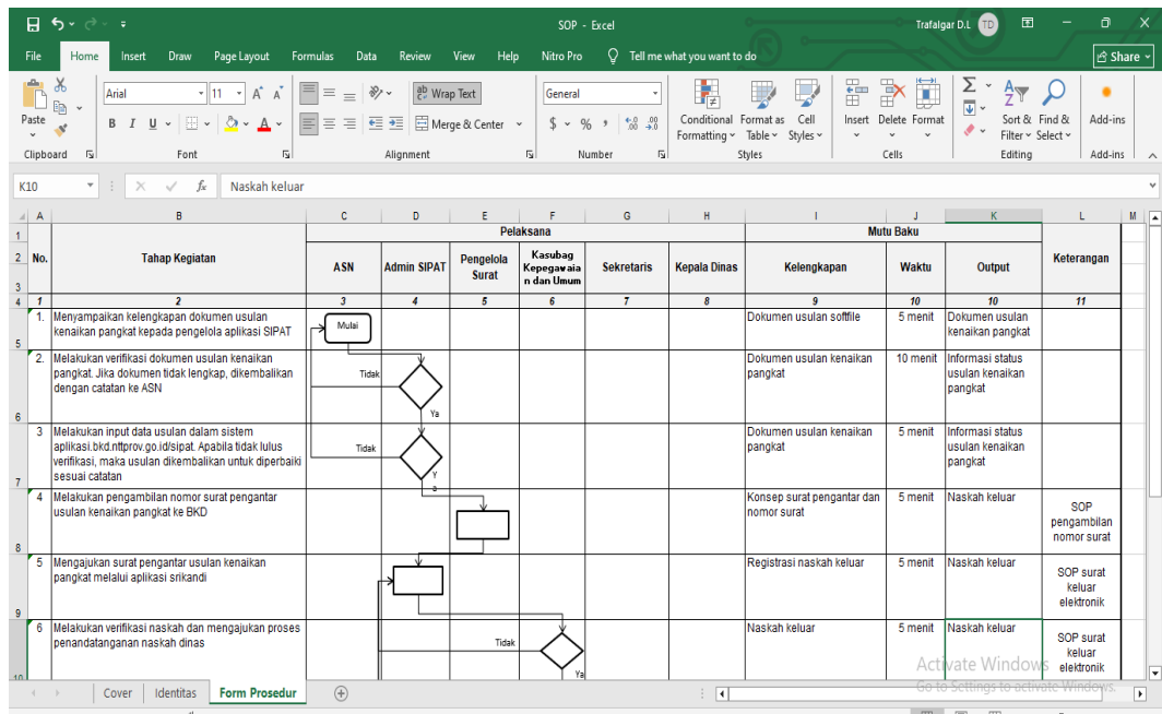
Gambar 11. Alur SOP
