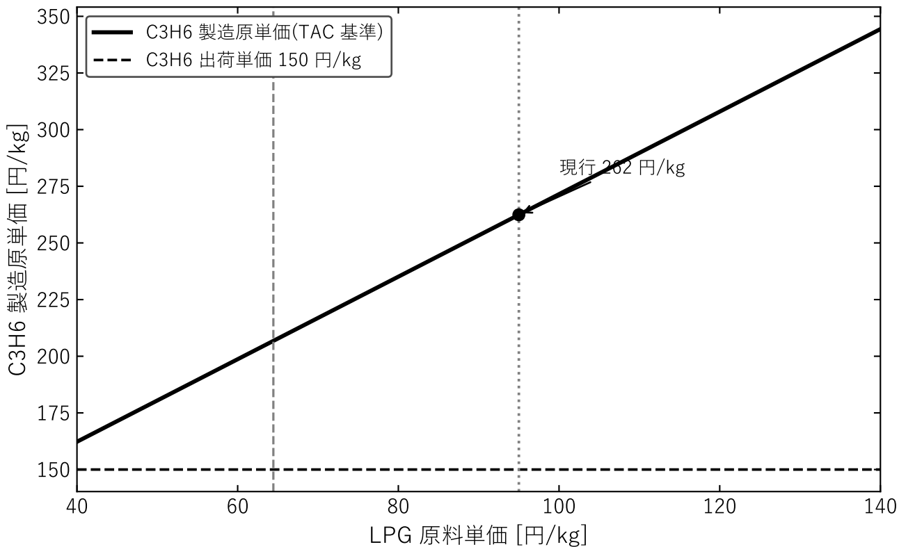
LPG 原料価格と C3H6 製造原単価(最適設計を固定)
