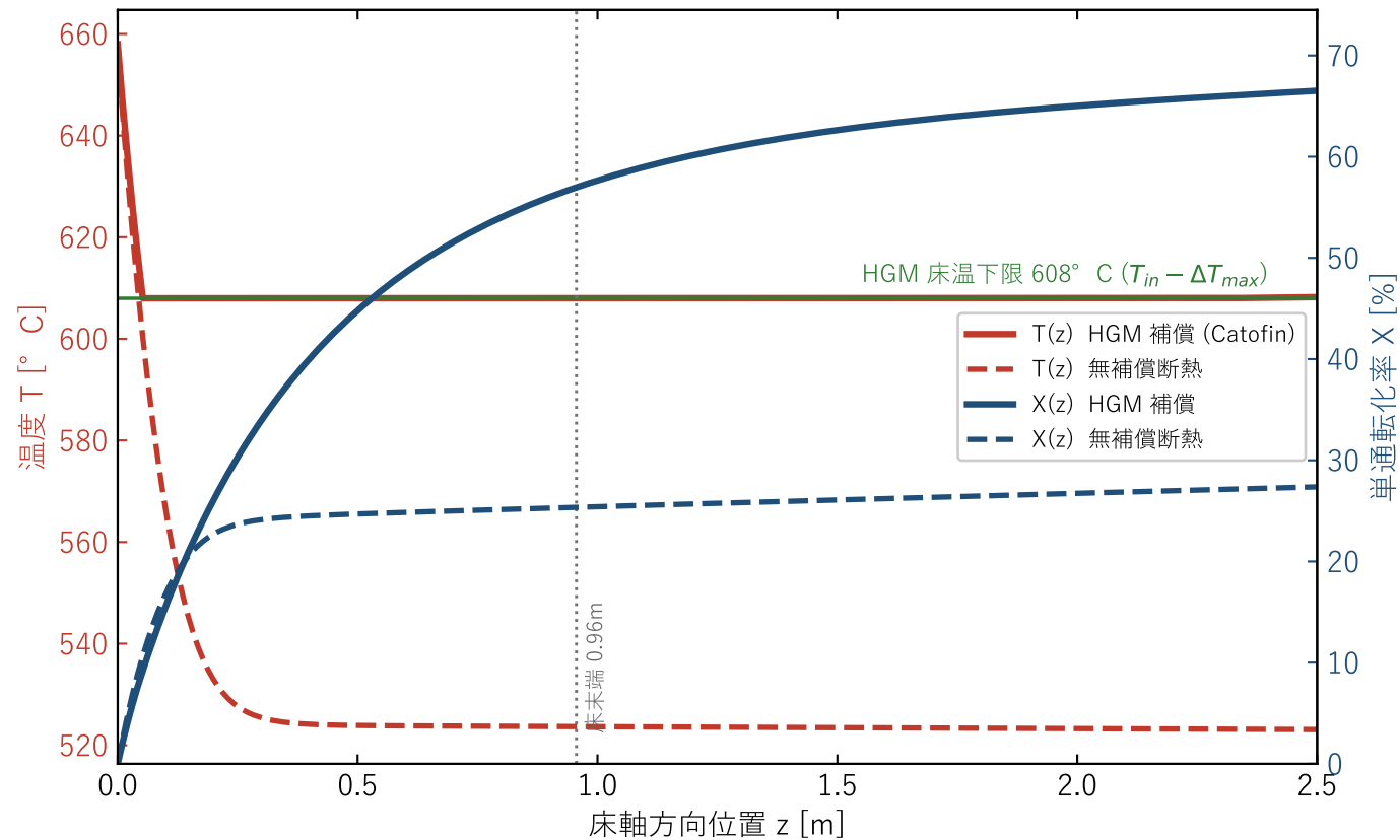
反応器内 軸方向プロファイル: HGM補償が床温を維持し転化率を伸ばす
