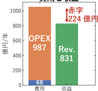
費用と収益
