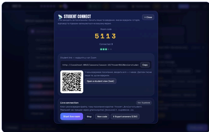
Панель Student connect: код кімнати, посилання, QR-код, статус з'єднання, експорт відповідей.
