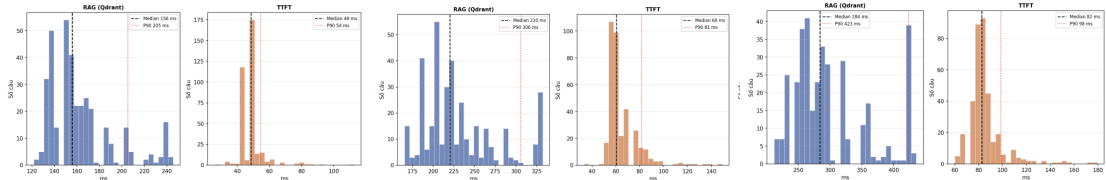
Hình 4.3: Phân bố thời gian RAG và thời gian sinh phần trả lời đầu tiên theo các cấu hình truy xuất
