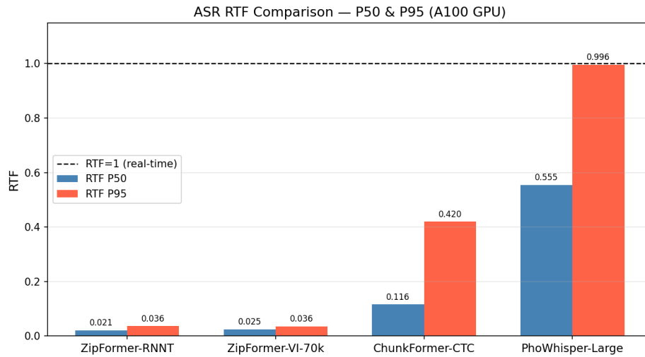
Hình 4.5: So sánh real-time factor của các mô hình ASR
