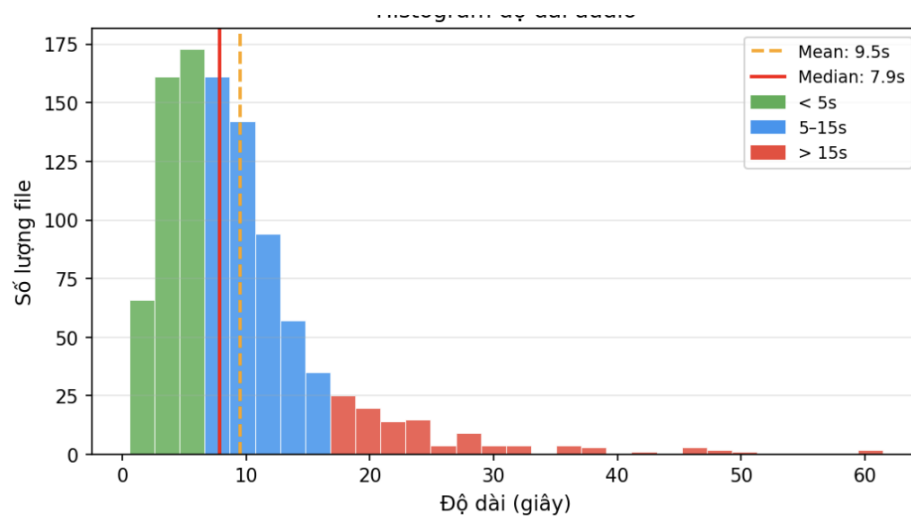
Hình 4.2: Phân bố độ dài audio trong tập đánh giá
