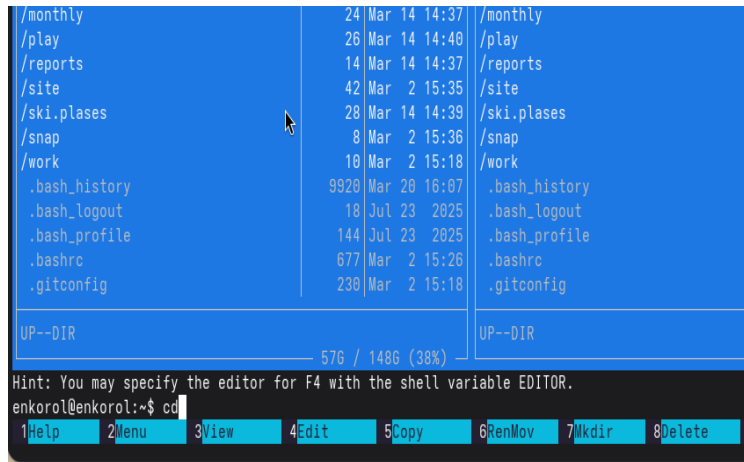
Рисунок 16: Переход в домашний каталог
