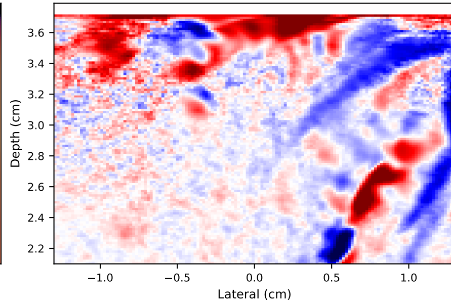
Color Doppler (Kasai)
