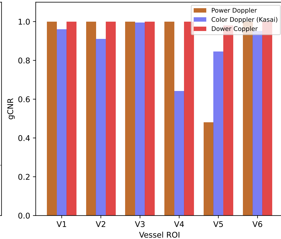
Magnitude gCNR
