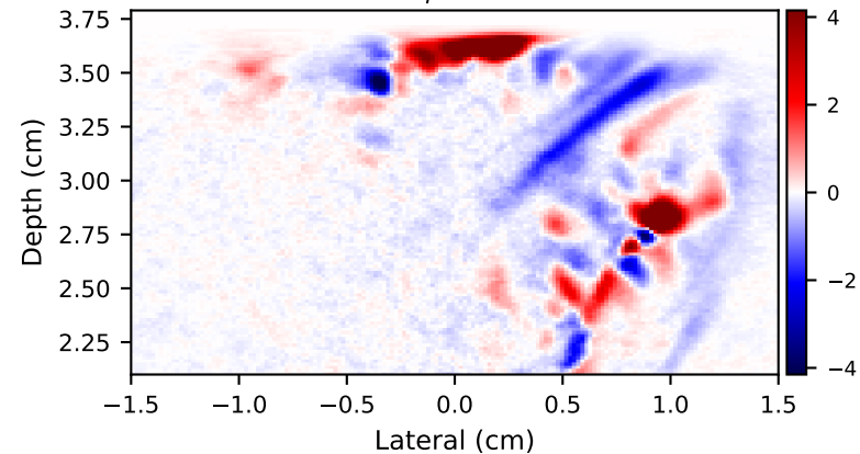
v_\phi \cdot G_R
