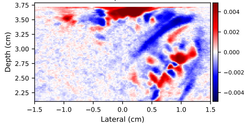
v_\phi \cdot R^2
