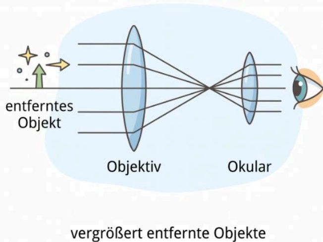
Fernrohr
