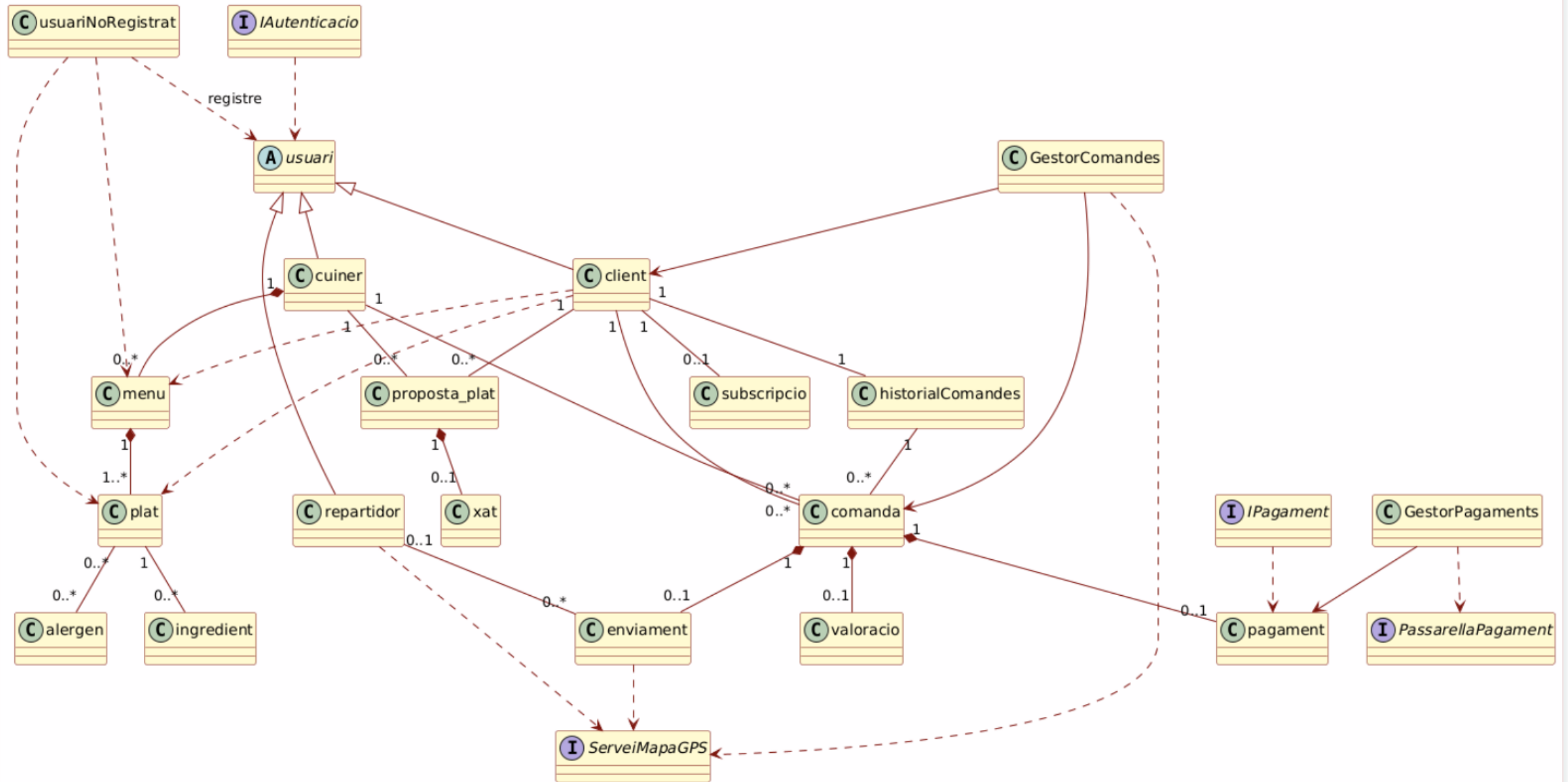
Diagrama de classes - QueMenges
