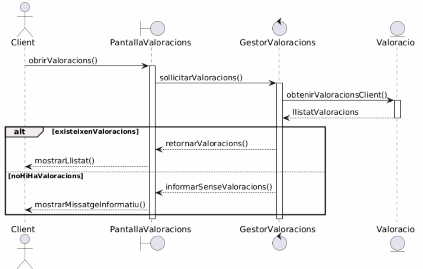
Diagrama de seqüència - Veure les meves valoracions
