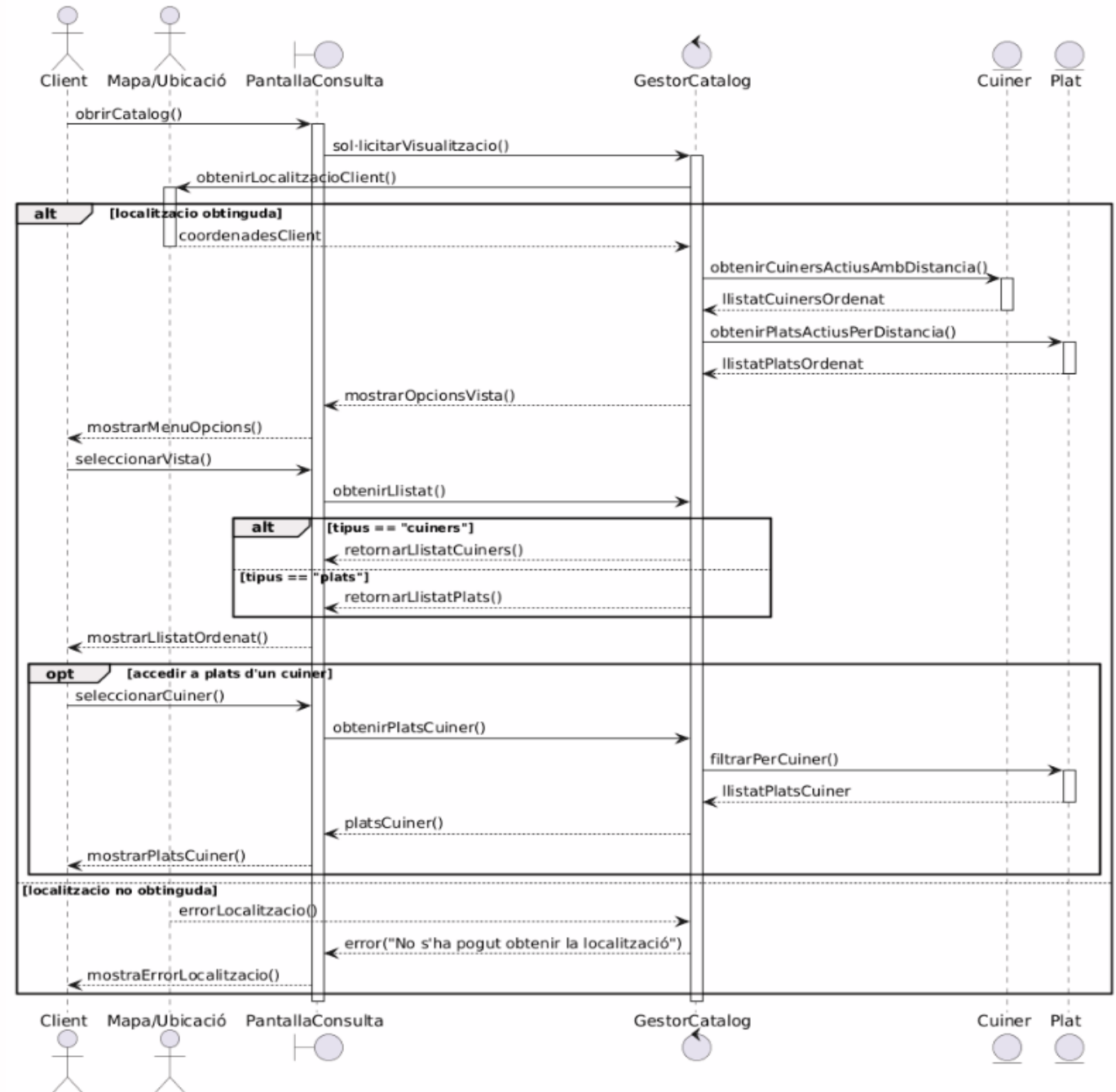
Diagrama de seqüència - Veure plats/menús o cuiners actius
