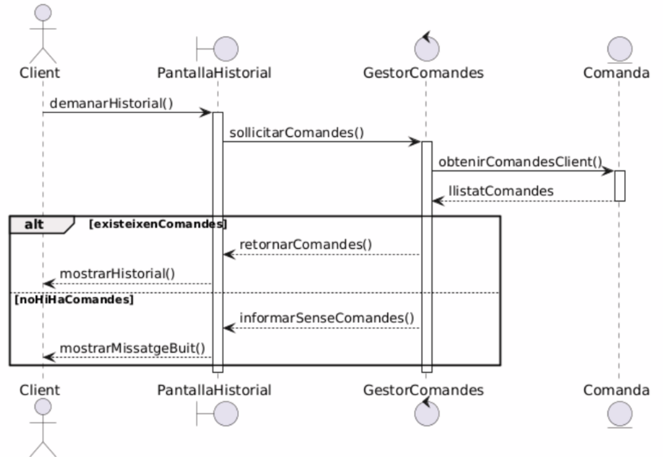
Diagrama de seqüència - Veure historial de comandes
