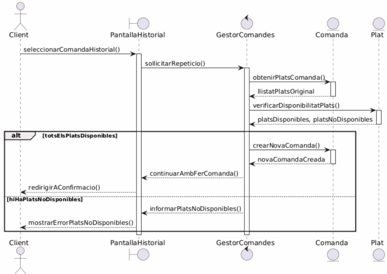
Diagrama de seqüència - Repetir una comanda anterior
