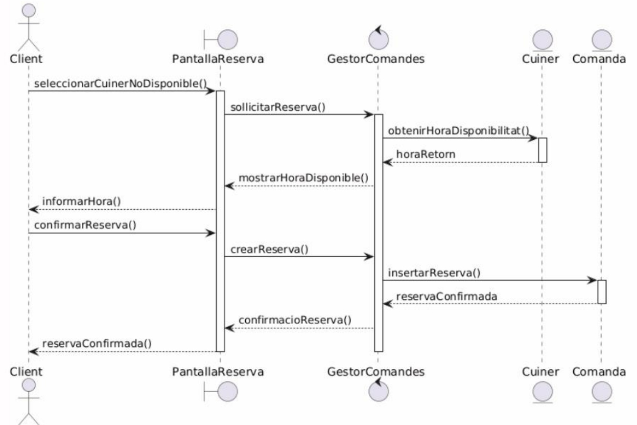
Diagrama de seqüència - Reservar comanda (cuiner no disponible)
