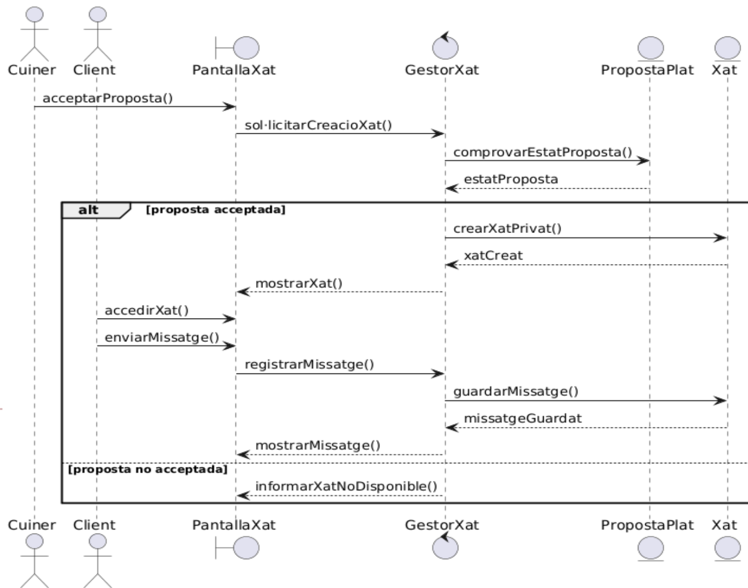
Diagrama de seqüència - Xat amb el cuiner
