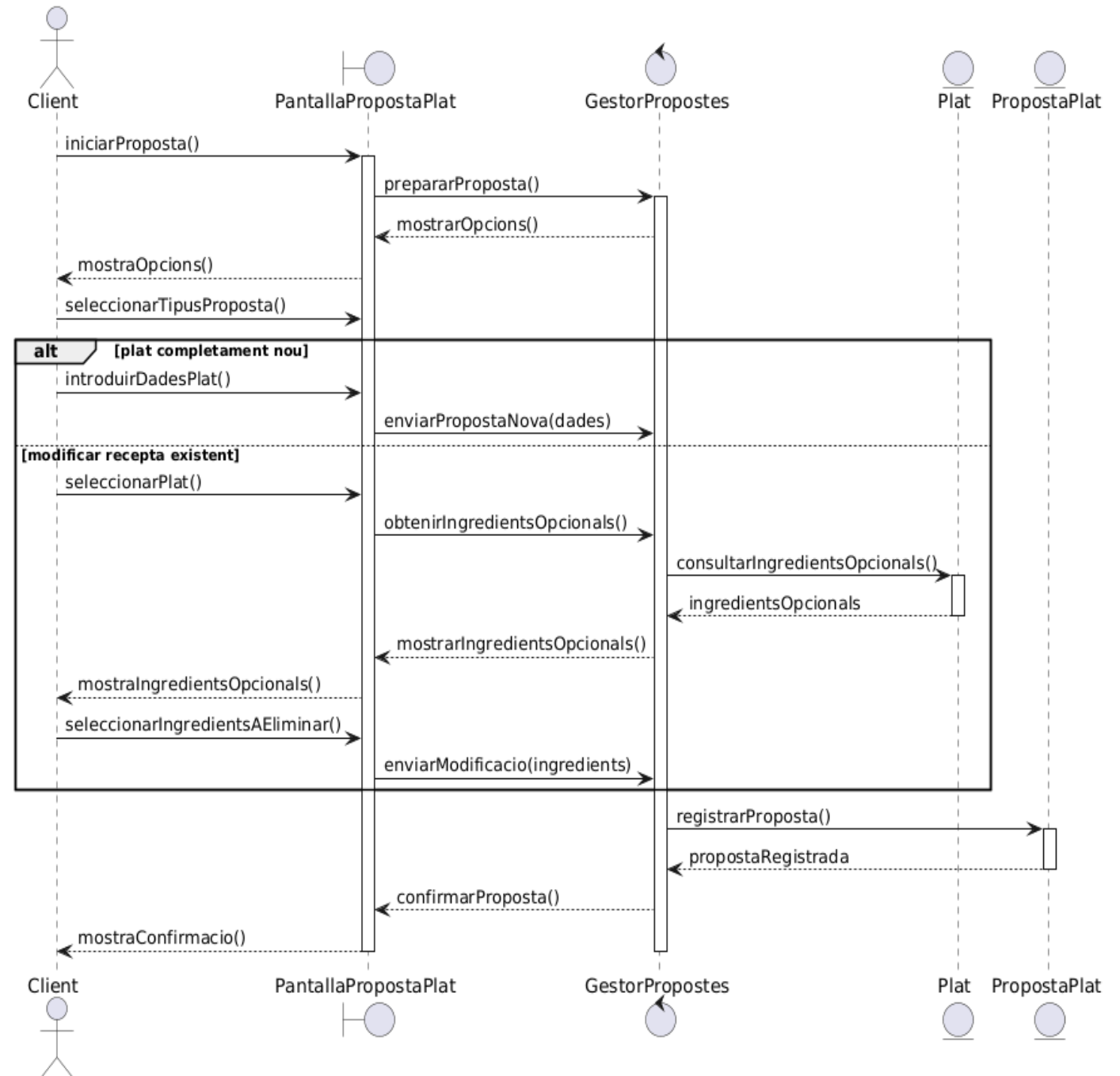
Diagrama de sequencia - Proposar un plat personalitzat
