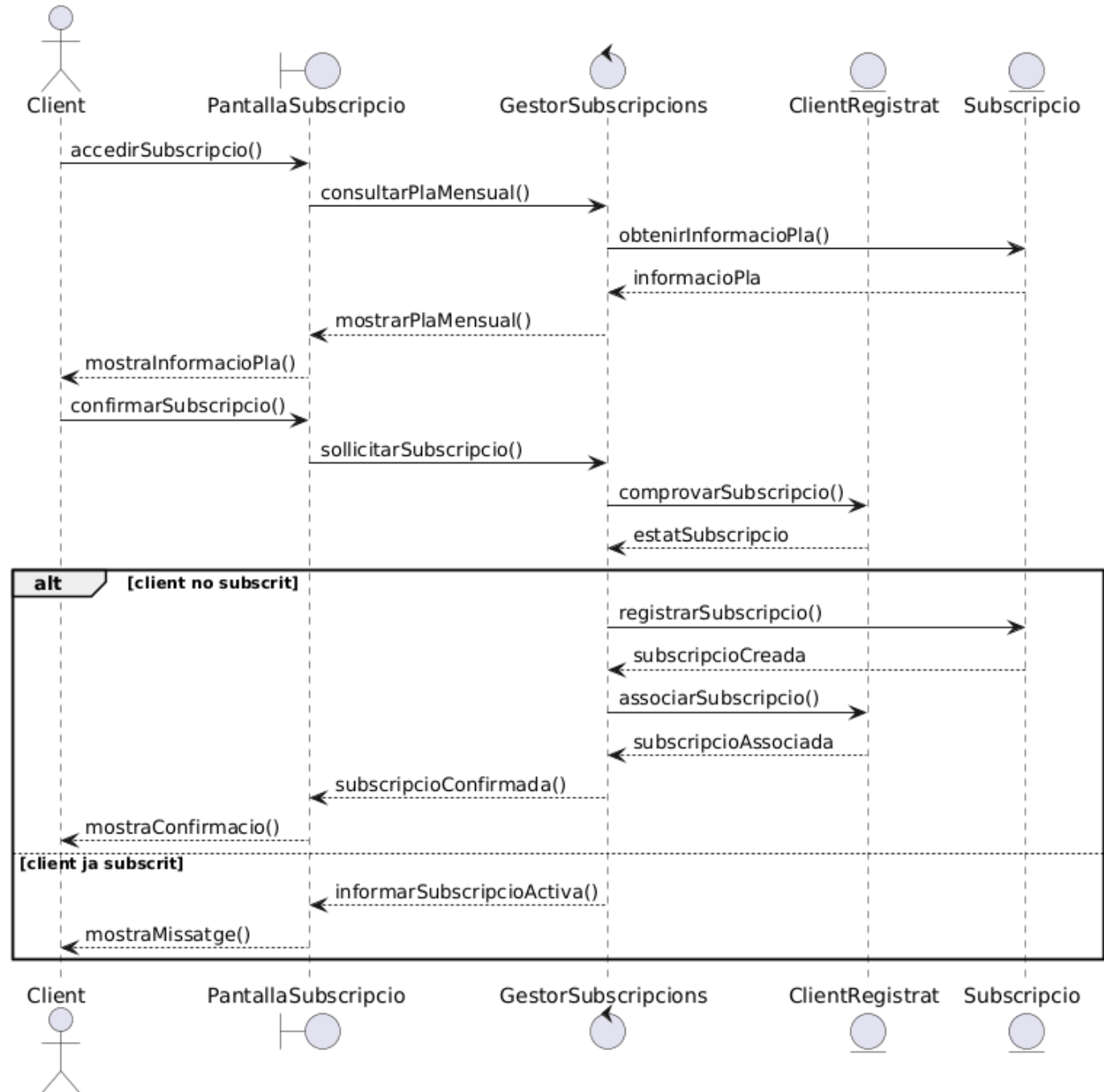
Diagrama de sequencia - Subscriure's a un pla mensual
