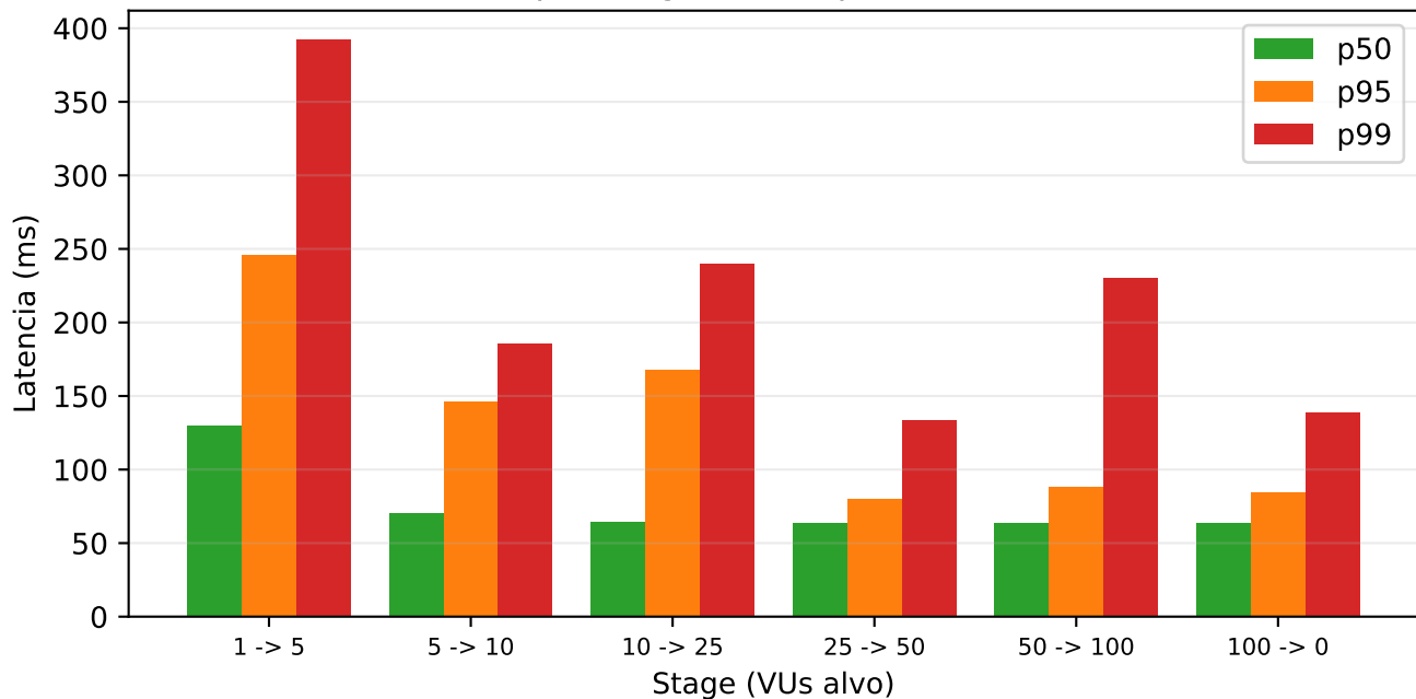
Latencia por stage da rampa de concorrência
