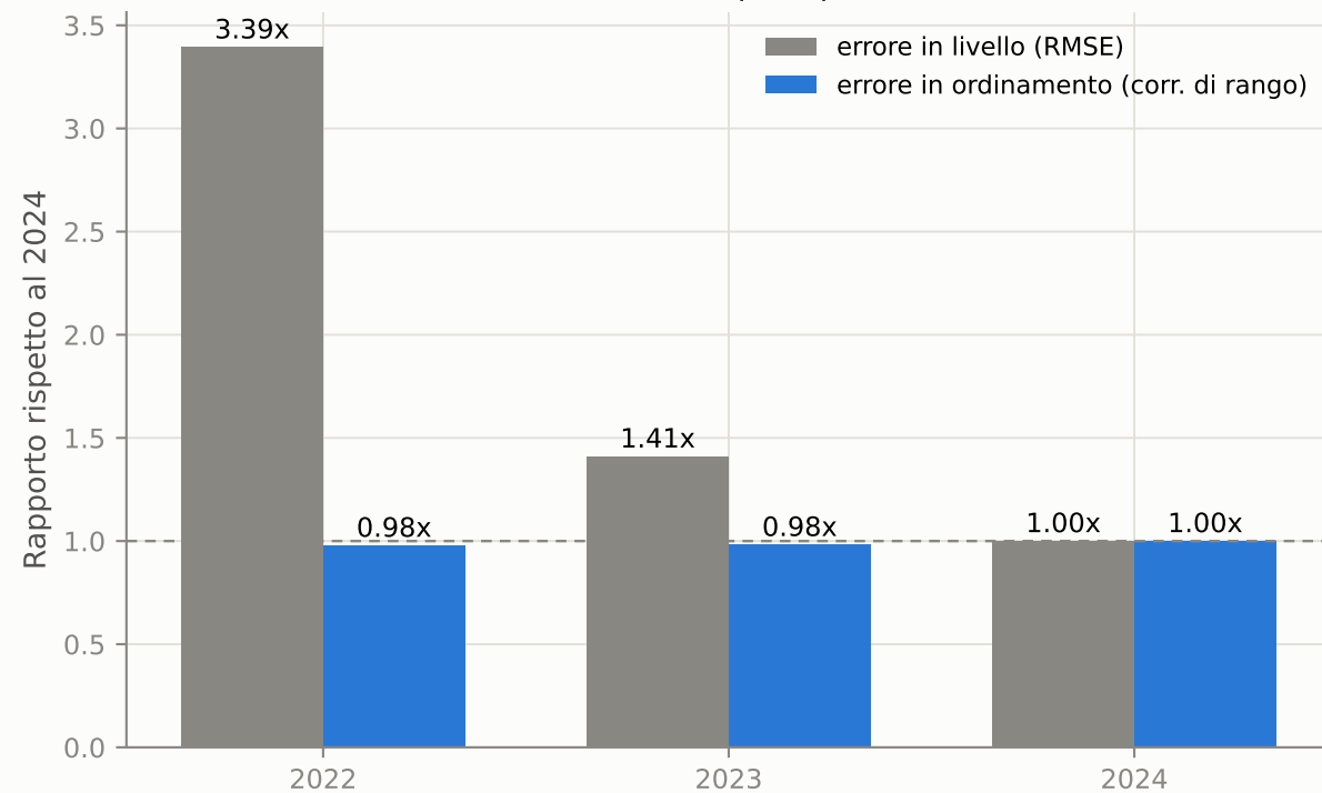
L'errore in livello cambia di un fattore tre, l'ordinamento quasi per nulla
