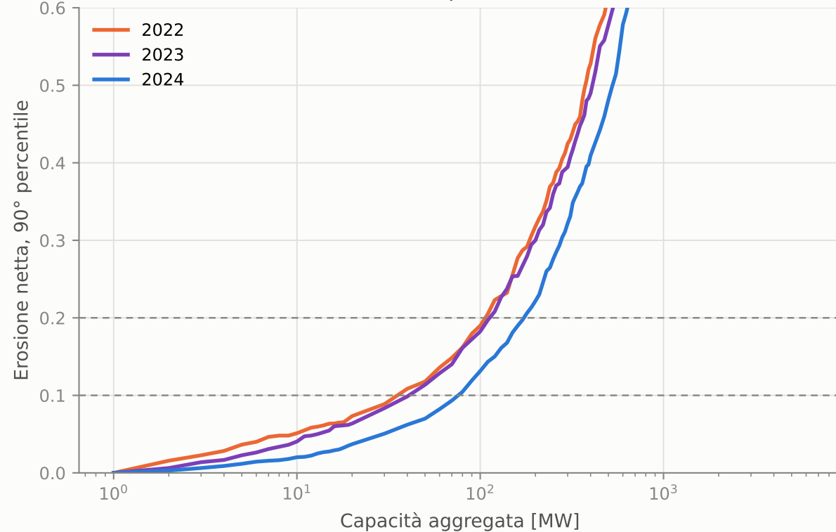
Le curve intere, non solo le soglie: l'ordinamento non dipende dal livello scelto
