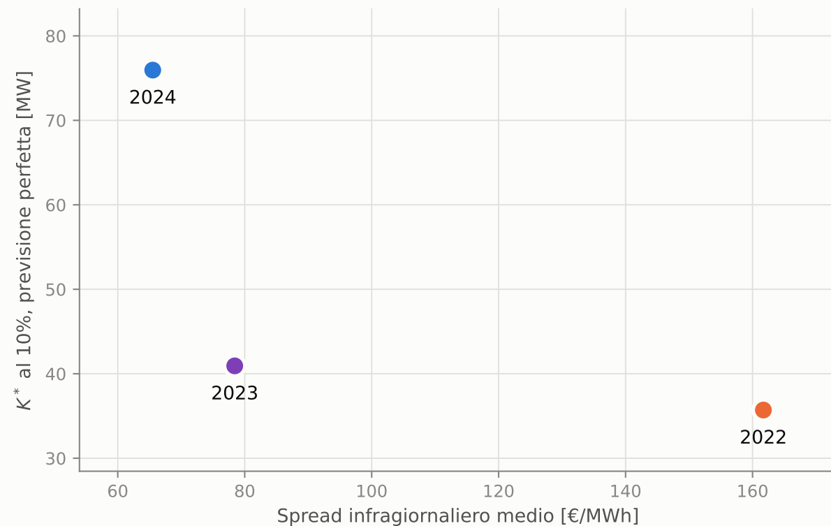
L'errore in livello cambia di un fattore tre, l'ordinamento quasi per nulla
