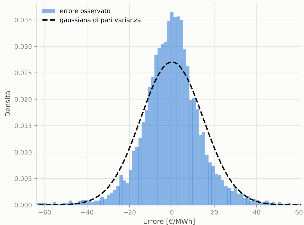
Curtosi in eccesso +3.97: più massa al centro e nelle code, meno nelle spalle
