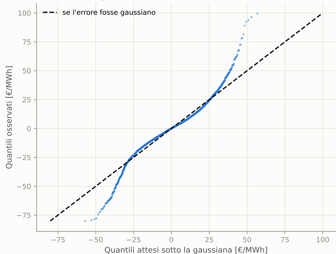
Le code osservate escono dalla retta: gli errori estremi sono molto più frequenti
