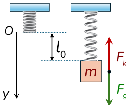
Figura 1.7: Sistema masa-muelle en la posición de equilibrio con las dos fuerzas que intervienen. El eje y apunta en sentido positivo hacia abajo.
