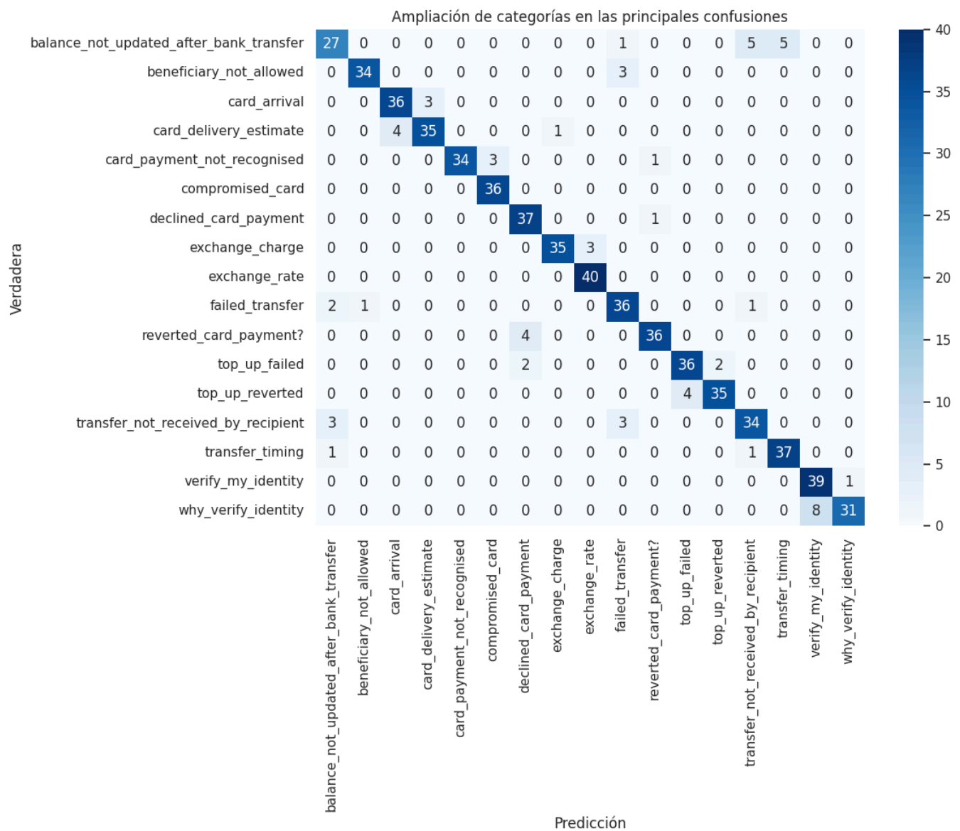
Figura 7. Ampliación de las principales categorías confundidas.
