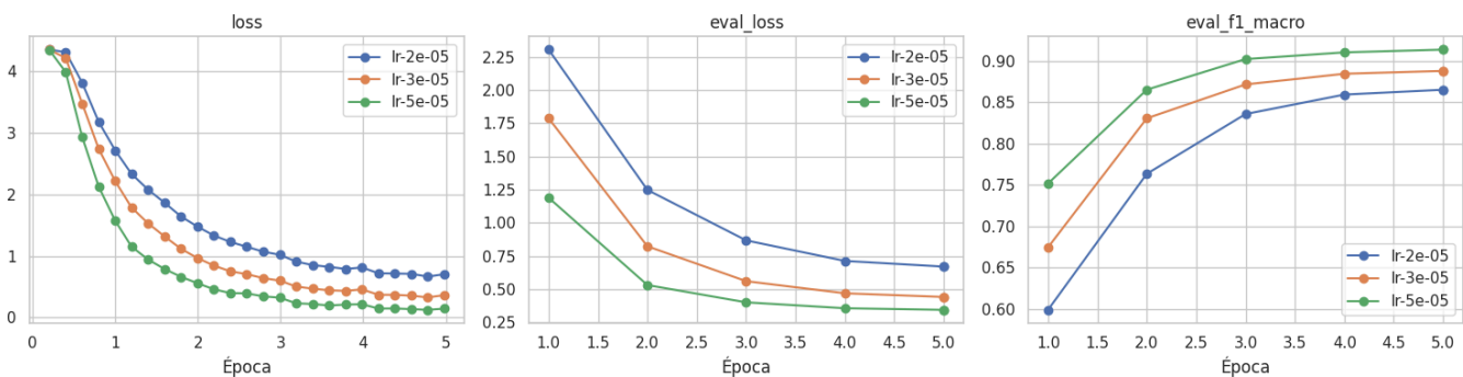
Figura 4. Curvas de entrenamiento y validación de las tres tasas de aprendizaje.
