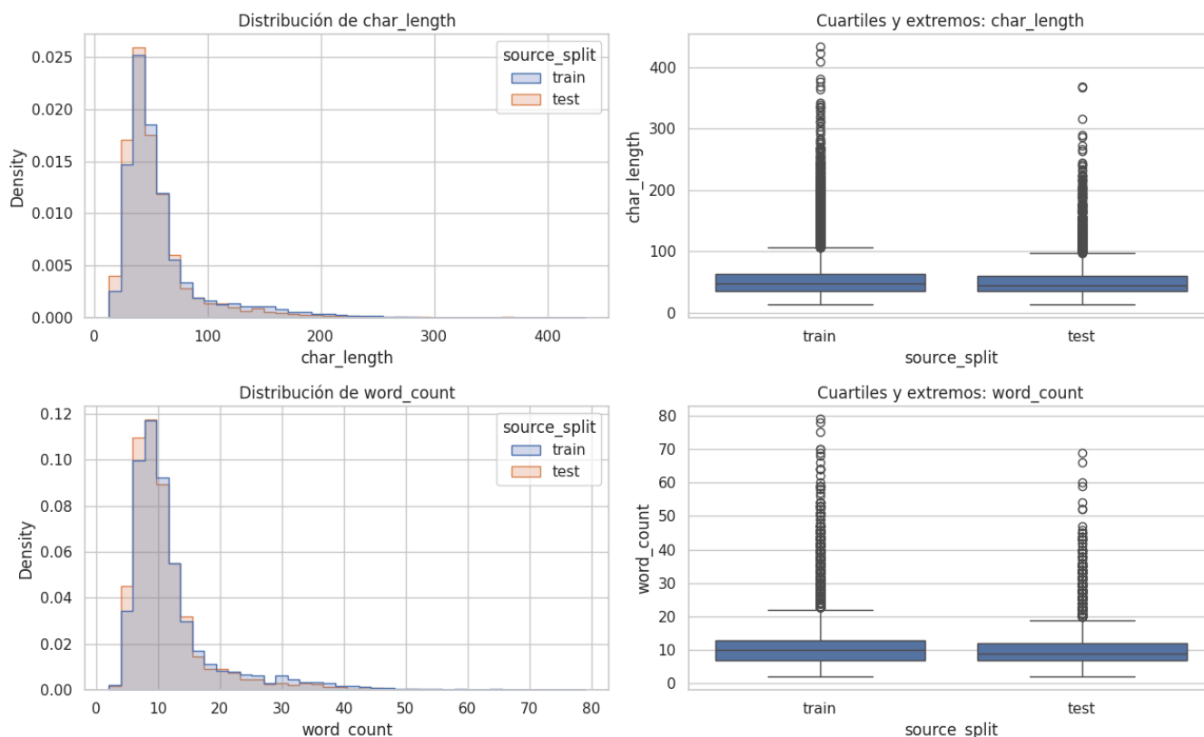
Figura 1. Longitud en caracteres y número de palabras por partición.
