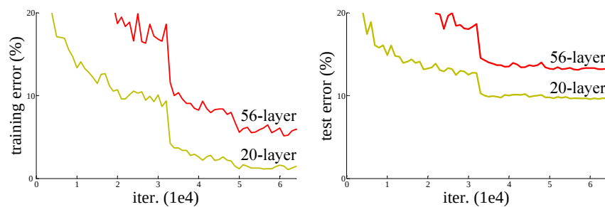
Figura 38 – Desempenho de duas redes neurais não residuais com 56 e 20 camadas. A esquerda a taxa de erro durante o treinamento, a direita a taxa de erro em relação ao conjunto de testes.
