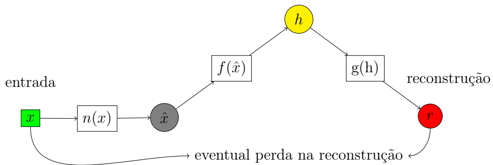
Figura 36 – Representação funcional de um denoising autoencoder : Sendo o vetor x uma entrada e n uma função que adiciona um ruído aleatório então a informação com ruído \hat{x} é definida como \hat{x} = n(x) , portanto o vetor h é resultado da aplicação de uma função codificadora f sobre \hat{x} : h = f(\hat{x}) , finalmente r é a reconstrução de x a partir de h através de uma função decodificadora g : r = g(h) . É importante notar que r é comparada com x e não com \hat{x} .
