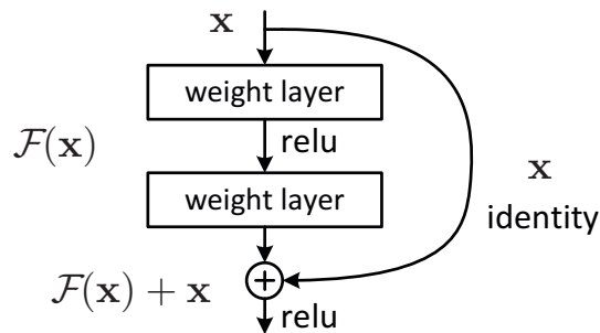
Figura 29 – Bloco Residual: x contorna as camadas intermediárias F(x) via uma função identidade somando-se a própria F(x) ao final do bloco.
