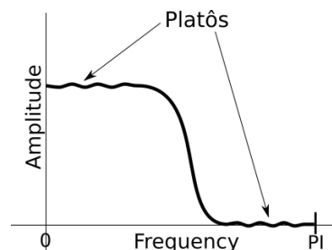
Figura 6 – Platôs não maximamente planos de um filtro digital: características de outros filtros wavelet , distintos da família de Daubechies
