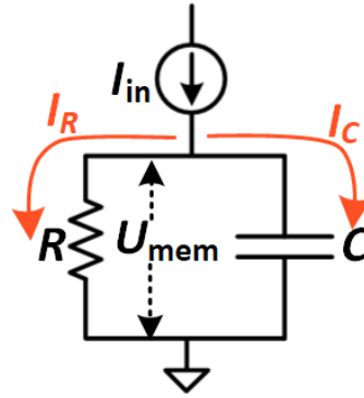
Figura 21 – Modelo RC para correntes: I_{in} = I_R + I_C
