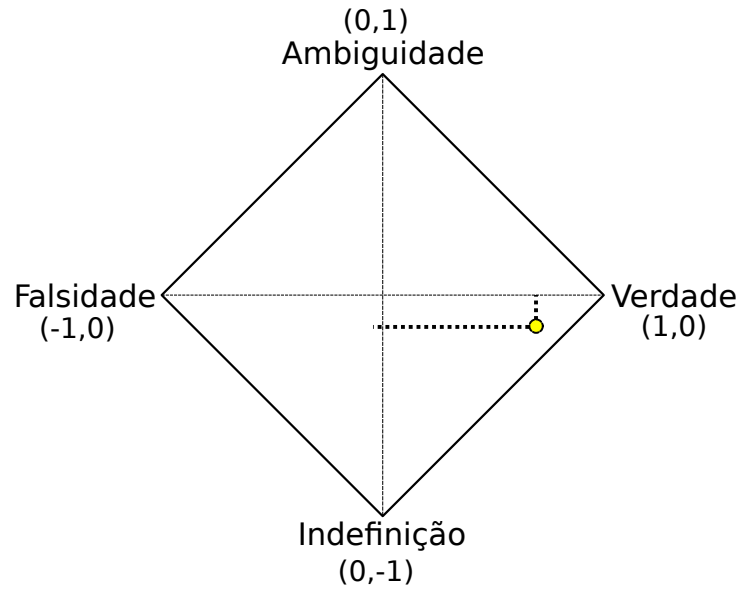
Figura 9 – O plano paraconsistente: O pequeno círculo indica os graus de falsidade(-1,0), verdade(1,0), indefinição(0,-1) e ambiguidade(0,1)
