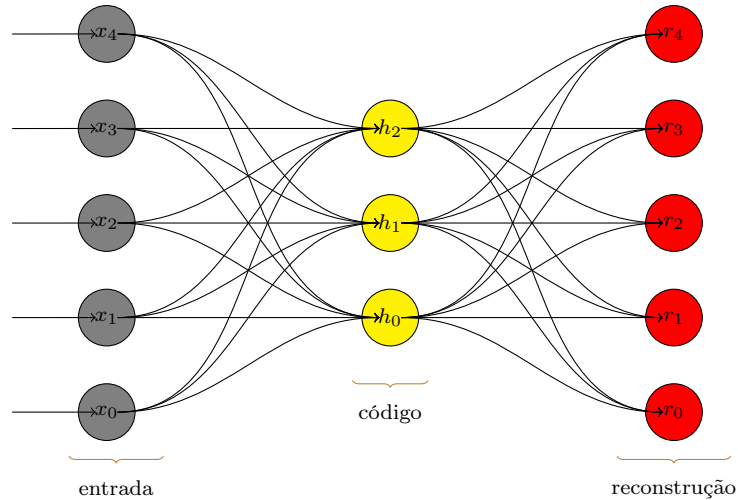
Figura 26 – Exemplo esquemático de um autoencoder sub-completo ou clássico: Os nós de entrada estão em cinza, a camada de código em amarelo contém as características codificadas e finalmente a camada de reconstrução em vermelho contém uma cópia aproximada da entrada.
