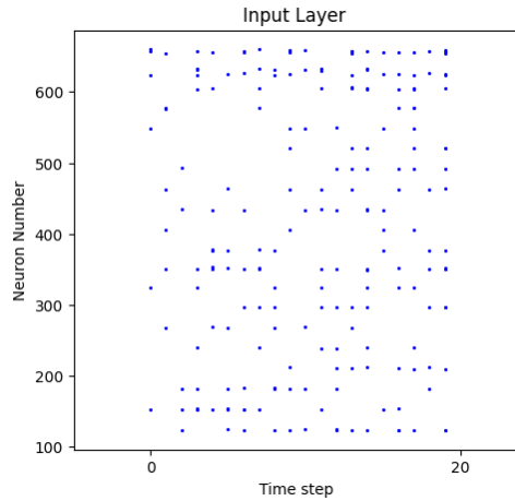
Figura 20 – Atividade dispersa de uma RNP: O eixo horizontal representa o momento no qual os dados estão sendo processados e o vertical representa o número do neurônio (índice) na RNP. Note que, na maior parte do tempo, muito poucos neurônios são ativados.
