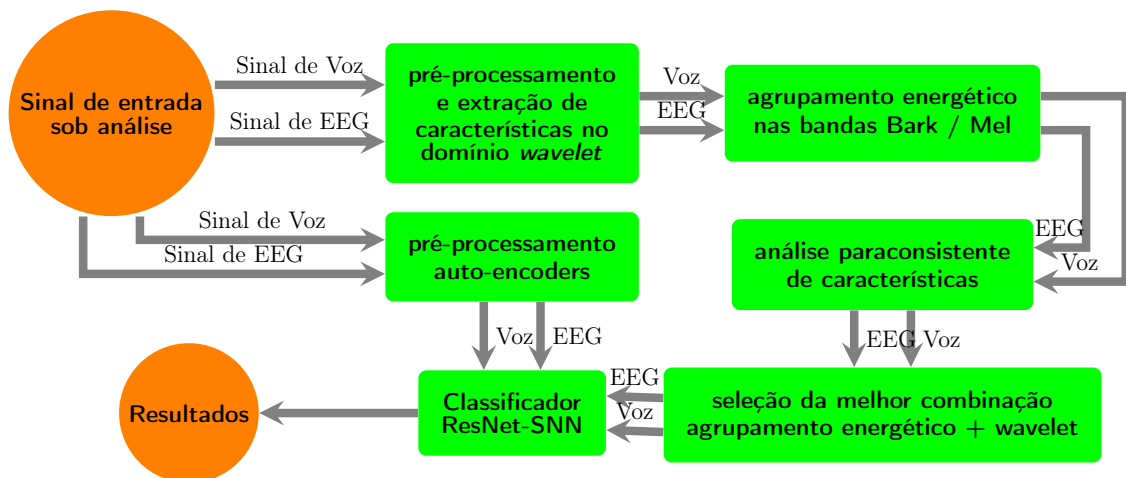
Figura 33 – Fluxograma da estratégia proposta
