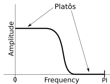
Figura 5 – Platôs maximamente planos em um filtro digital: característica da família de Daubechies
