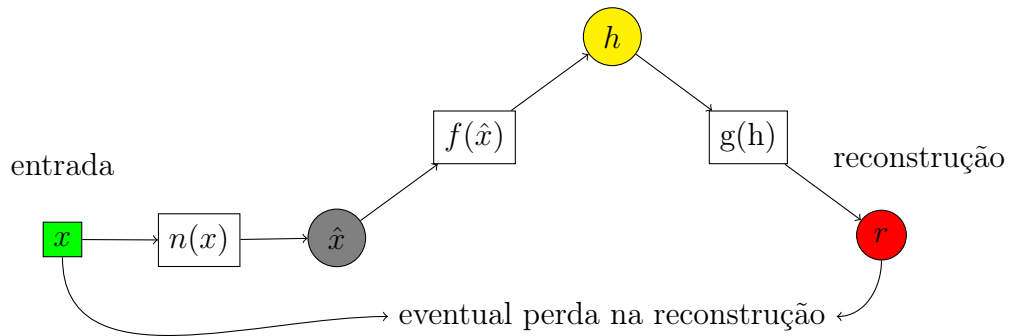
Figura 28 – Representação funcional de um denoising autoencoder : Sendo o vetor x uma entrada e n uma função que adiciona um ruído aleatório então a informação com ruído \hat{x} é definida como \hat{x} = n(x) , portanto o vetor h é resultado da aplicação de uma função codificadora f sobre \hat{x} : h = f(\hat{x}) , finalmente r é a reconstrução de x a partir de h através de uma função decodificadora g : r = g(h) . É importante notar que r é comparada com x e não com \hat{x} .
