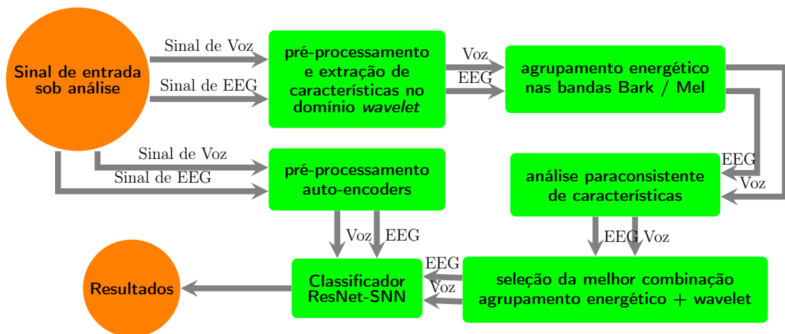
Figura 36 – Fluxograma da estratégia proposta
