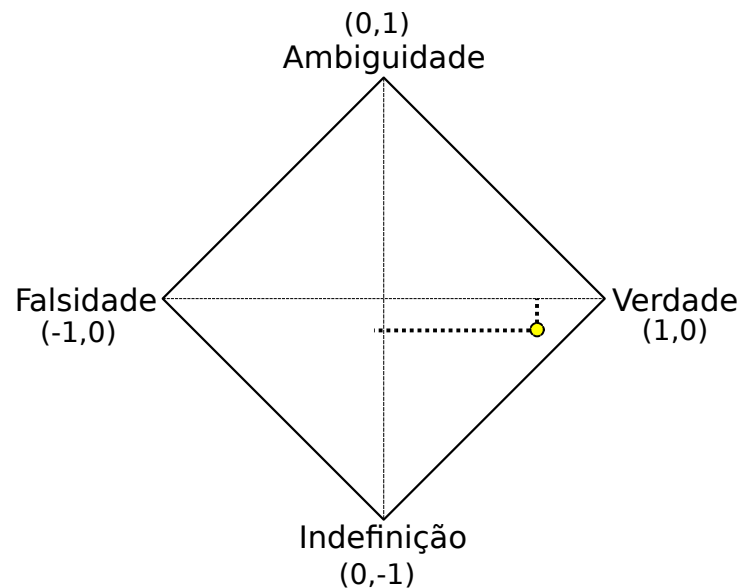
Figura 12 – O plano paraconsistente: O pequeno círculo indica os graus de falsidade(-1,0), verdade(1,0), indefinição(0,-1) e ambiguidade(0,1)
