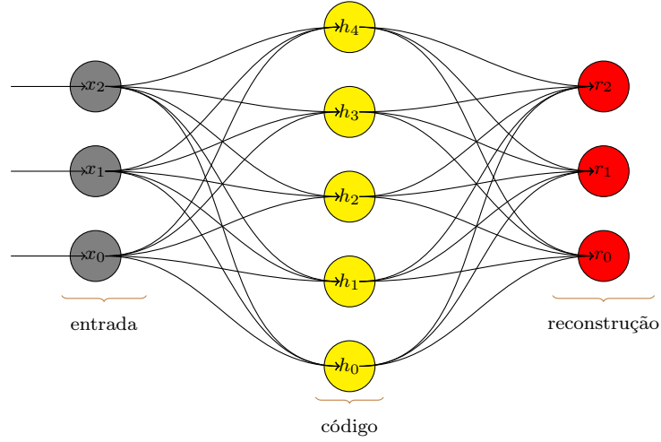
Figura 30 – Exemplo esquemático de um autoencoder supra-completo.
