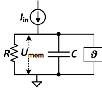
Figura 21 – O modelo RC
