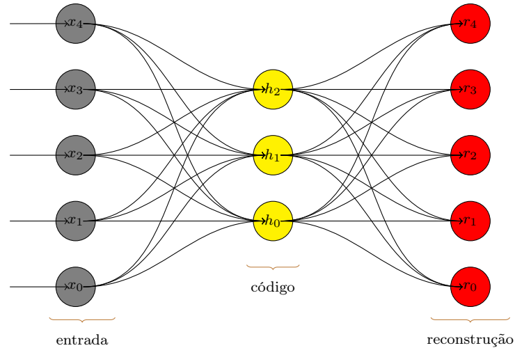
Figura 29 – Exemplo esquemático de um autoencoder sub-completo ou clássico: Os nós de entrada estão em cinza, a camada de código em amarelo contém as características codificadas e finalmente a camada de reconstrução em vermelho contém uma cópia aproximada da entrada.
