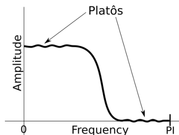
Figura 9 – Platôs não maximamente planos de um filtro digital: características de outros filtros wavelet , distintos da família de Daubechies
