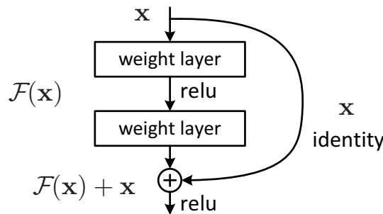
Figura 32 – Bloco Residual: x contorna as camadas intermediárias F(x) via uma função identidade somando-se a própria F(x) ao final do bloco.
