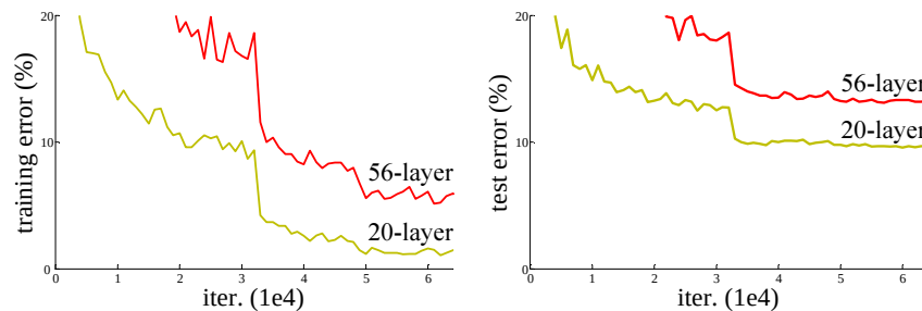
Figura 33 – Desempenho de duas redes neurais não residuais com 56 e 20 camadas. A esquerda a taxa de erro durante o treinamento, a direita a taxa de erro em relação ao conjunto de testes.
