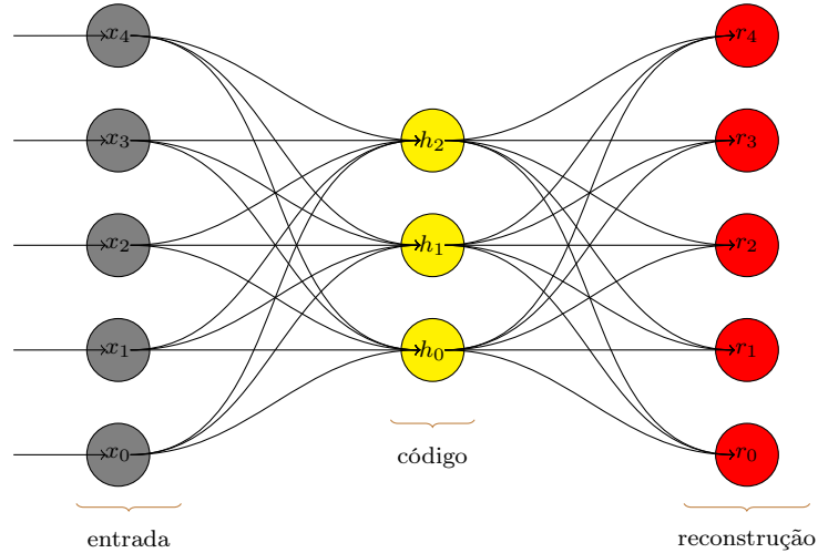
Figura 31 – Exemplo esquemático de um autoencoder sub-completo ou clássico: Os nós de entrada estão em cinza, a camada de código em amarelo contém as características codificadas e finalmente a camada de reconstrução em vermelho contém uma cópia aproximada da entrada.
