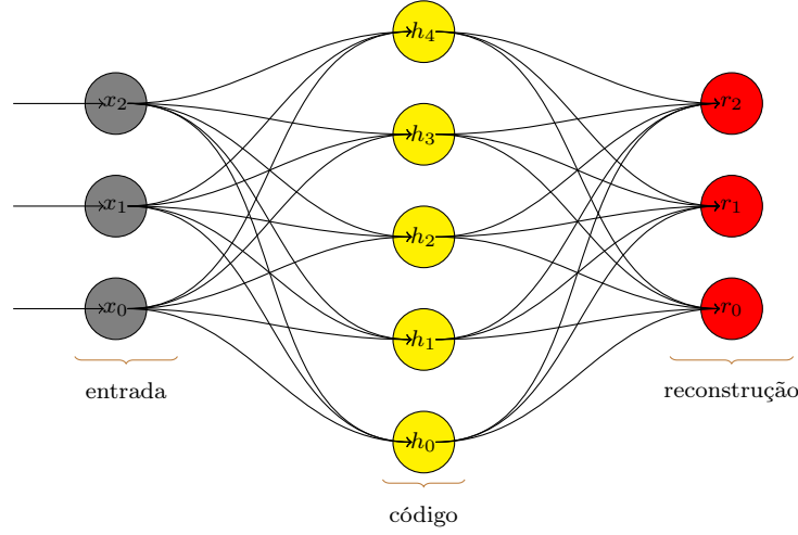
Figura 32 – Exemplo esquemático de um autoencoder supra-completo.
