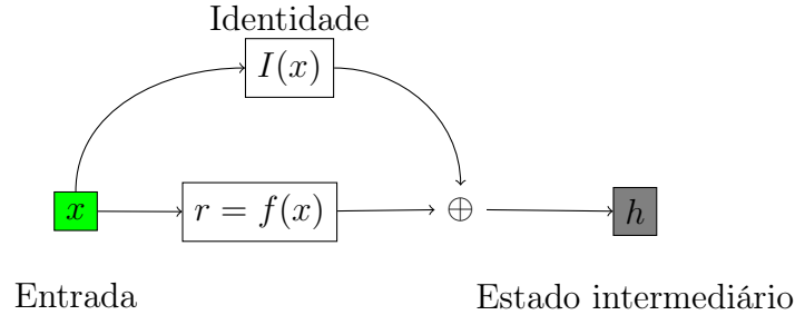
Figura 36 – Obtenção do resíduo: Se x é um vetor de entrada na rede e I(\cdot) é uma função identidade cujo valor é diretamente somado \oplus com o resultado produzido pelas várias camadas representadas por f(\cdot) , h é um vetor representando um estado intermediário de uma rede neural.
