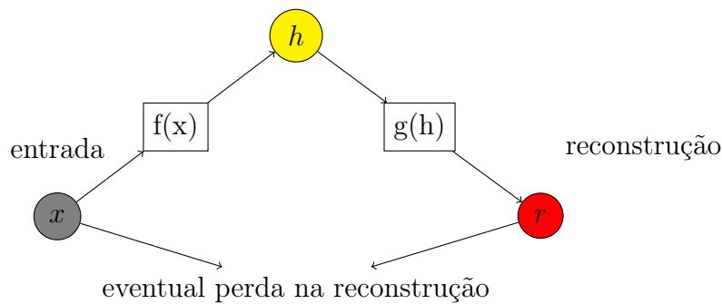
Figura 30 – Representação funcional de um autoencoder : Sendo o vetor x uma entrada, então o vetor h é estado resultante da aplicação de uma função codificadora f sobre x : h = f(x) , portanto r é a reconstrução de x a partir h através de uma função decodificadora g : r = g(h) . Tal processo pode ou não implicar em uma perda de informação.
