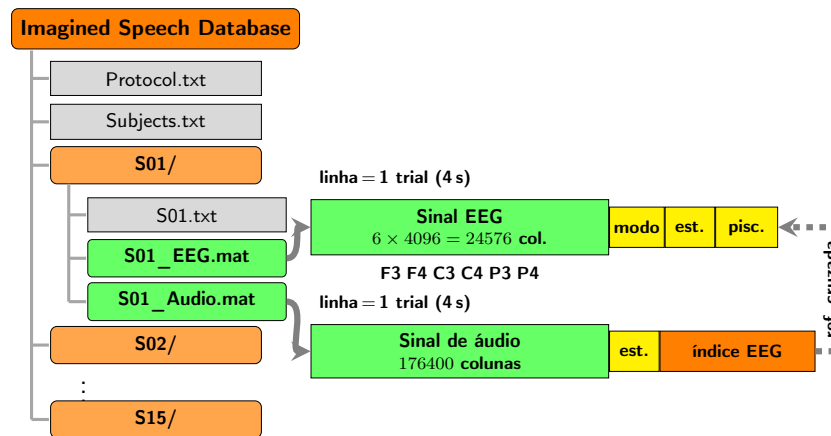
Figura 37 – Estrutura dos arquivos da base de sinais (CORETTO; GAREIS; RUFINER, 2017)
