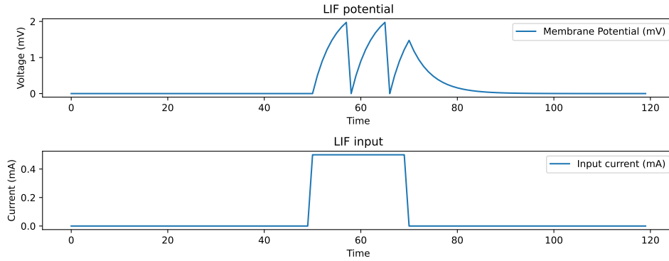
Figura 27 – Gráfico do LIF simulado completo: Foram fornecidos 0.5 mA de corrente no intervalo de tempo de 51 a 70.
