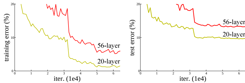
Figura 35 – Desempenho de duas redes neurais não residuais com 56 e 20 camadas. A esquerda a taxa de erro durante o treinamento, a direita a taxa de erro em relação ao conjunto de testes.
