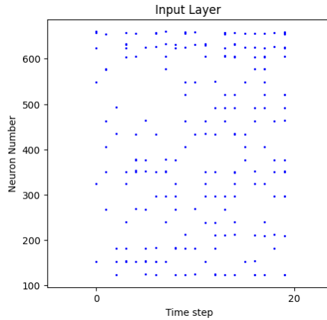
Figura 20 – Atividade dispersa de uma RNP: O eixo horizontal representa o momento no qual os dados estão sendo processados e o vertical representa o número do neurônio (índice) na RNP. Note que, na maior parte do tempo, muito poucos neurônios são ativados.
